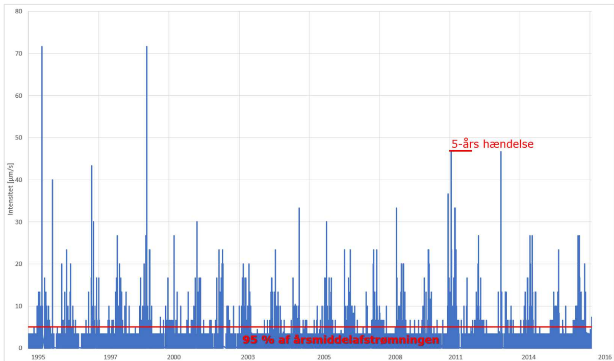
Figur 2 - Historisk regndata fra regnmåler ved Landbohøjskolen, der viser 95 % af årsafstrømningen og en 5-års hændelse.
