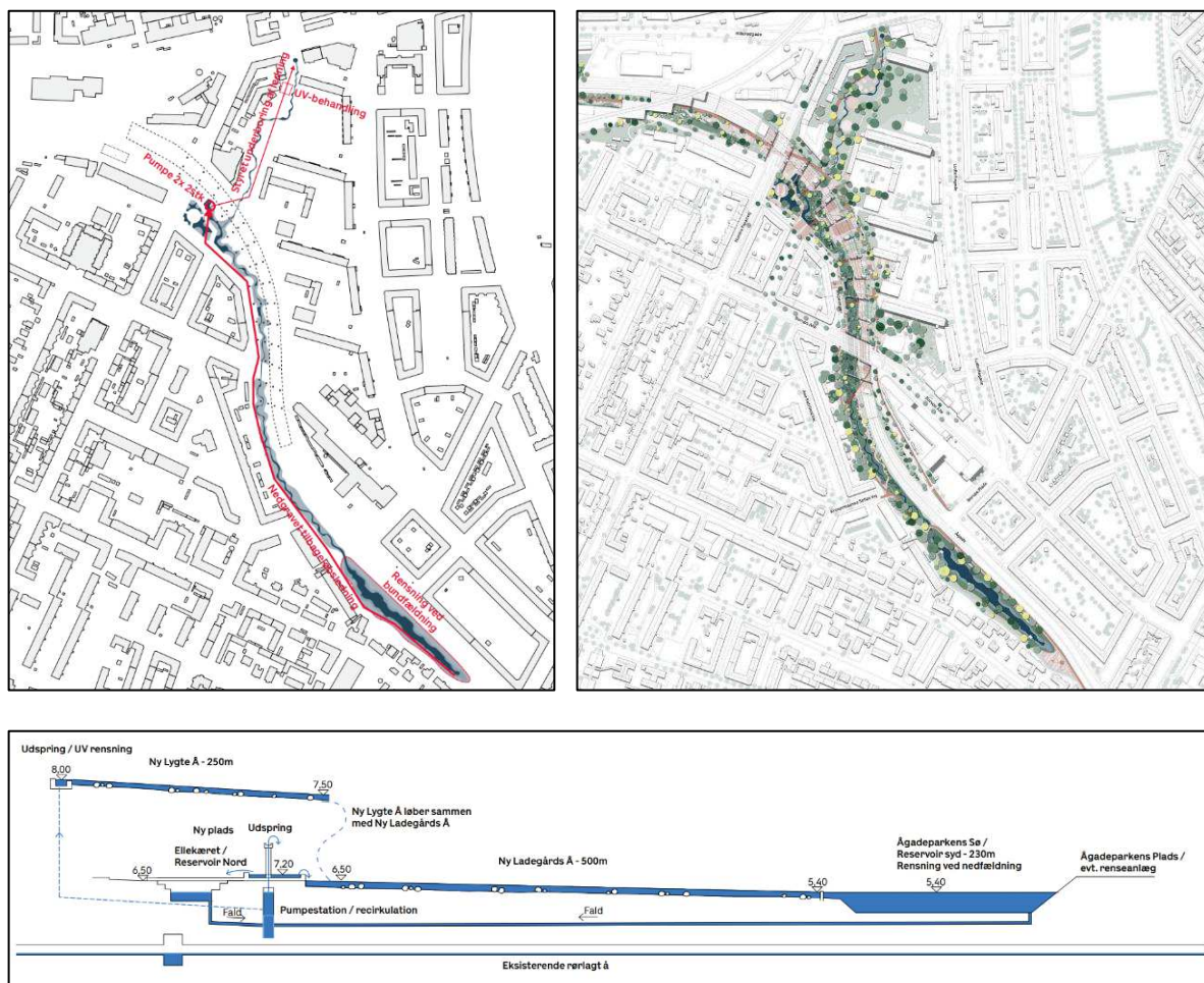
Figur 12 - Illustrationer fra Idéoplæg til omdannelse af Bispeengen [3]
