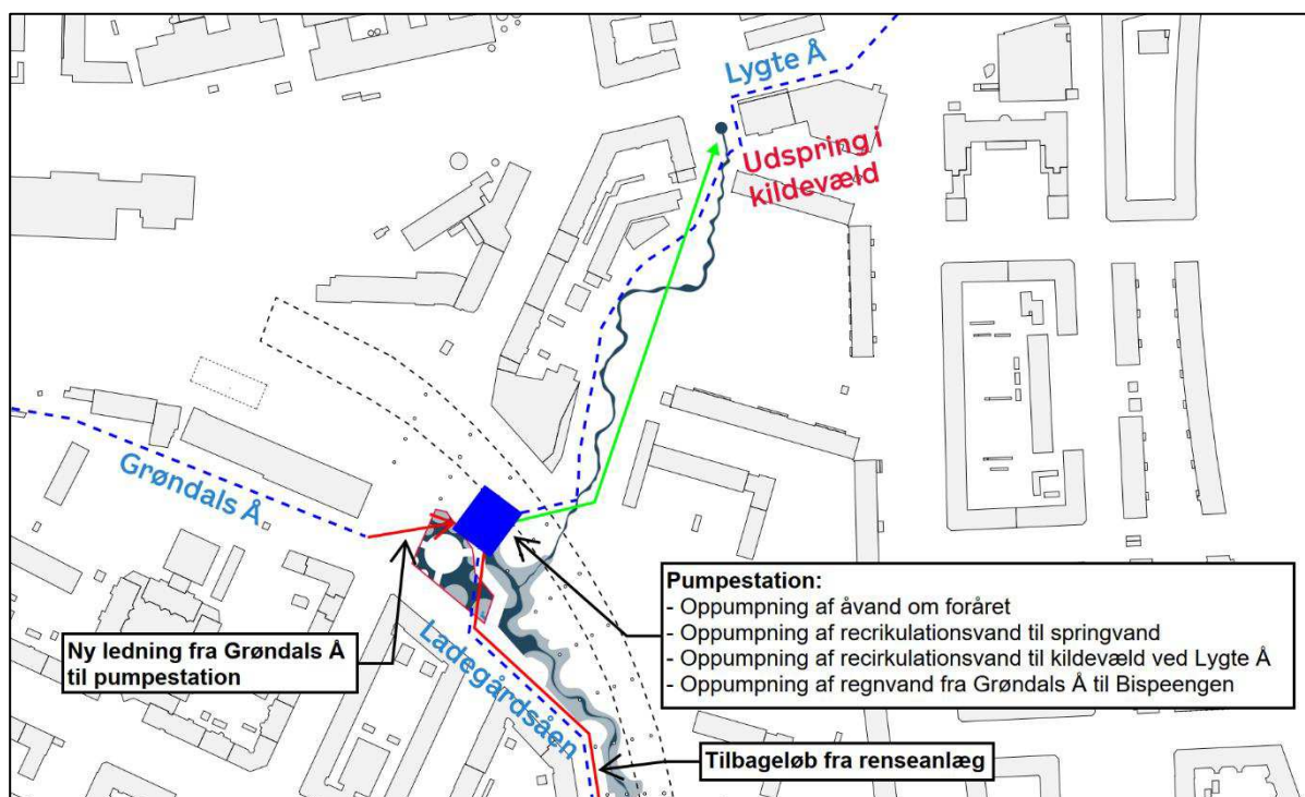
Figur 15 - Bispeengen-projekt med pumpe til recirkuleringsvand og de rørlagte vandløb inkl. ny tilslutning af Grøndals Å. Baggrundskortet er taget fra Idéoplægget til bispeengen [3].
