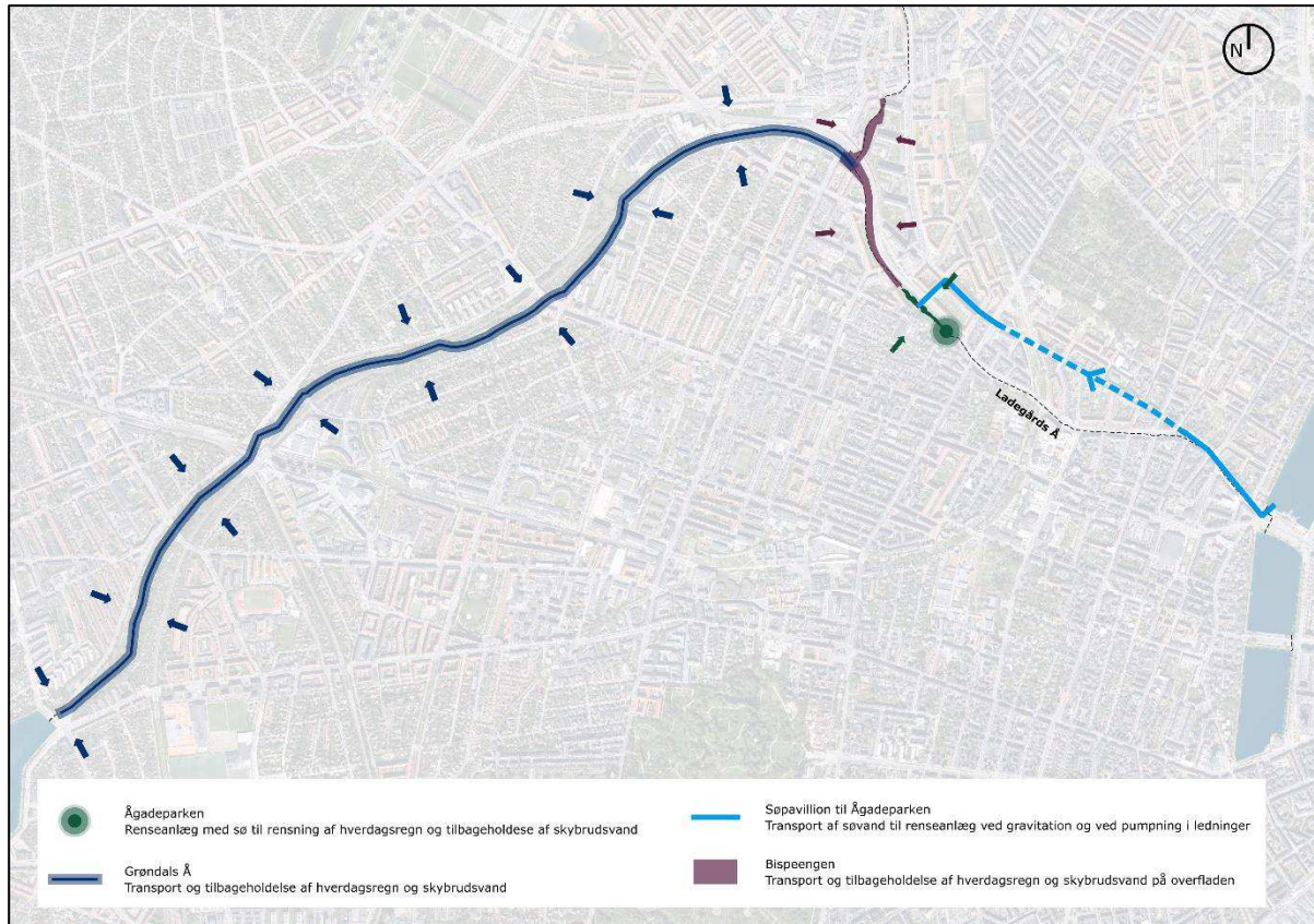
Figur 9 - Den fuldt udbyggede system med renseanlæg og rensesø i Ågadeparken med tilkobling af oplandene til Grøndals Å, Bispeengen og umiddelbare opland til Ågadeparken.
