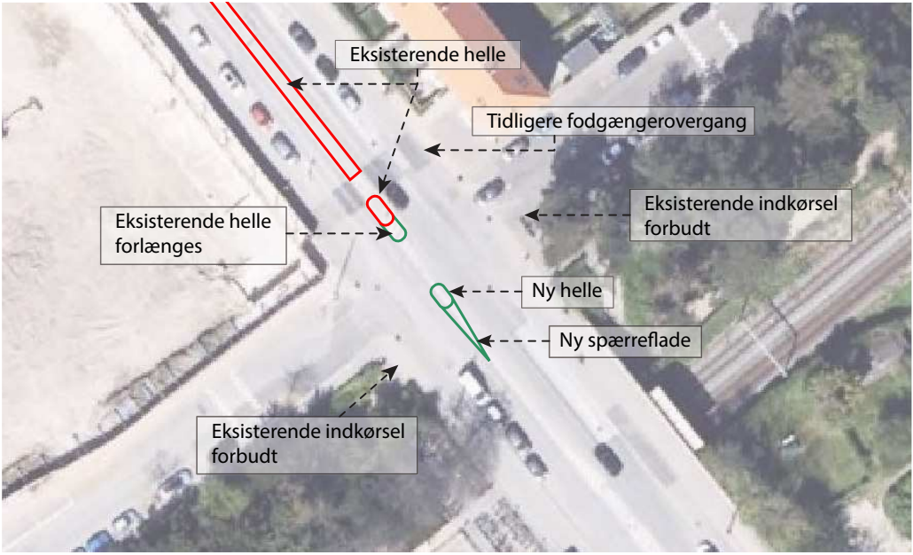
Figur 5-9 // Princip skitse for mere trafiksikker krydsning for cyklister af Godthåbsvej ved Grøndalsvænge Allé / Grøndals Parkvej. Kilde Danmarks Digitale Gadefoto 2023.
