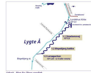
Udsnit - Plan for åbne vandløb
