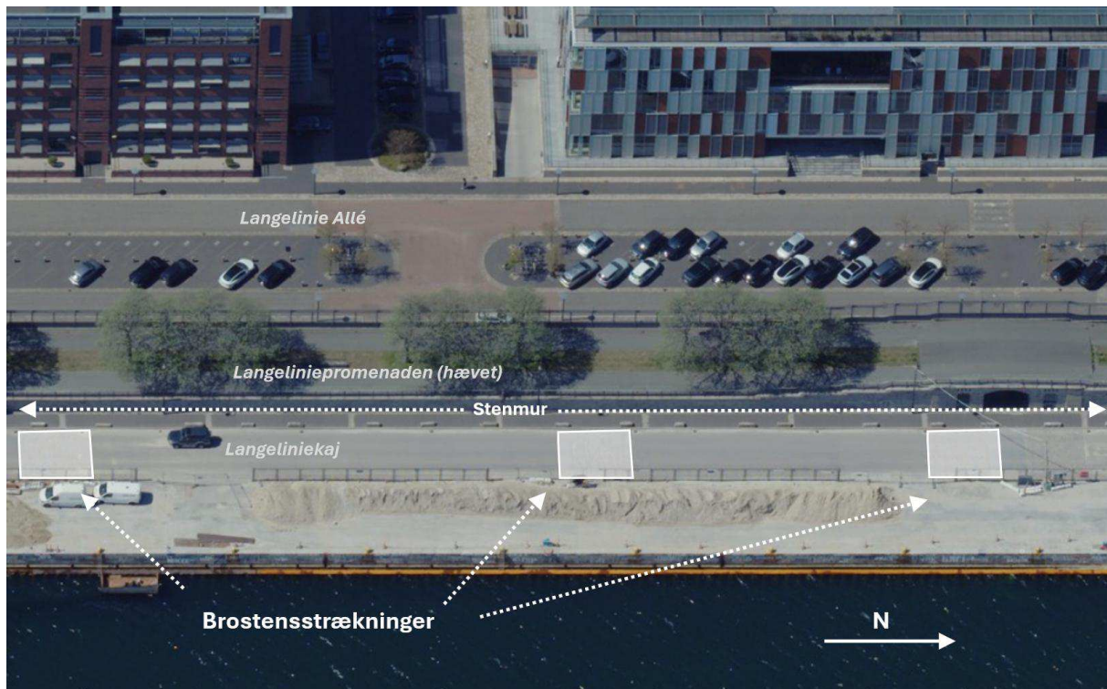
Figur 8-7. Udsnit af vejforløb på Langelinie kaj med angivelse af brostensstrækninger og stenmuren op imod promenaden. Skråfoto fra www.skraafoto.dataforsyningen.dk
