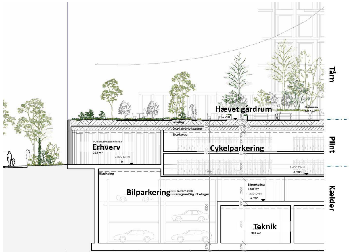
Figur 5-15. Principillustration af tværsnit gennem kælder og plint. III.: Lendager. 2025
