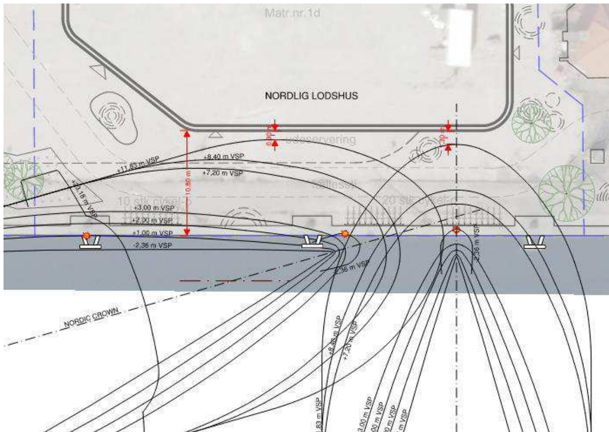
Figur 16-3. Nordligt Lodshus. Nordic Crown. Fendere sejles af og færge støder ind i betonkant med værste mulige vinkel til kaj. Situation til højre viser en frontal påsejling, hvor minimumsafstanden bliver ca. 1,3 m. Denne påsejling er kun teoretisk og ikke praktisk mulig. Situation til venstre viser en påsejling med den vinkel mellem færge og kaj, der giver den mindste afstand mellem færge og lodshus. Mindsteafstanden er her ca. 0,9 m.
