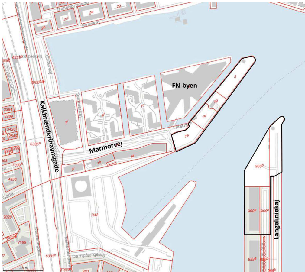
Figur 5-2. Projektets placering på de to molespidser ved indsejlingen til Møllebassin Frihavnen. Kort fra Danmarks Miljøportal
