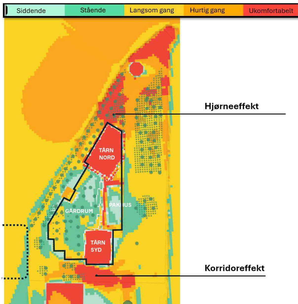
Figur 13-5. Resultat af vindanalyse af byggefelt på Langelinie. Placering af udlæg til mulig mobil badezone markeret med stiptet linje. Lenda-ger, 2026.
