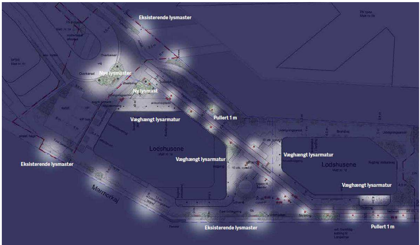
Figur 7-5. Belysningsplan for byggefelter på Marmormolen. III.: VLA, 2025.
