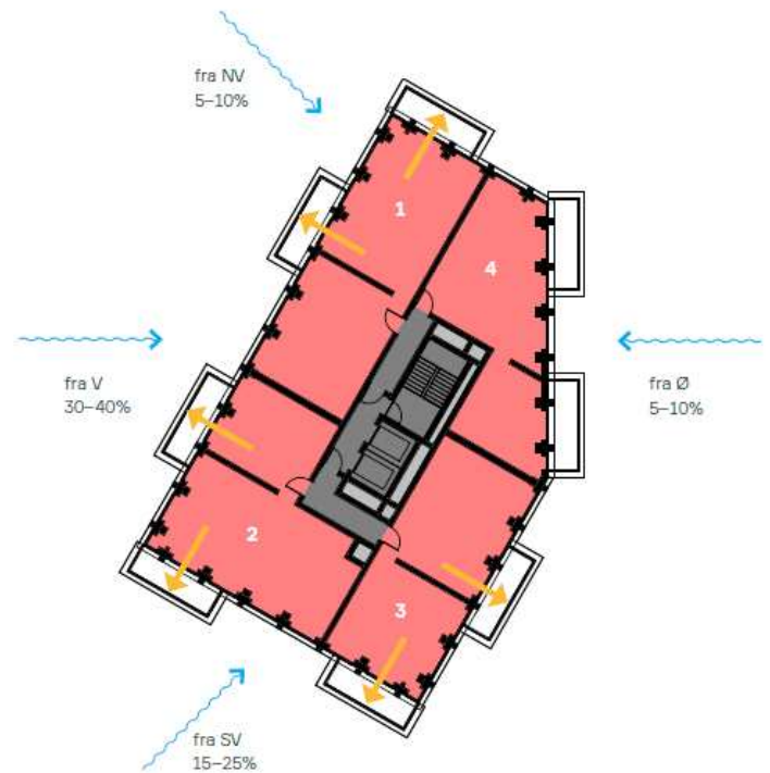
Figur 9-9. Disponering af altaner i to rytmer, der skifter fra etage til etage. Vindretningernes hyppighed angivet med procenttal. Pile inde fra lejligheder angiver mulighed for at tilgå altaner mod to verdenshjørner. Lendager, 2026.
