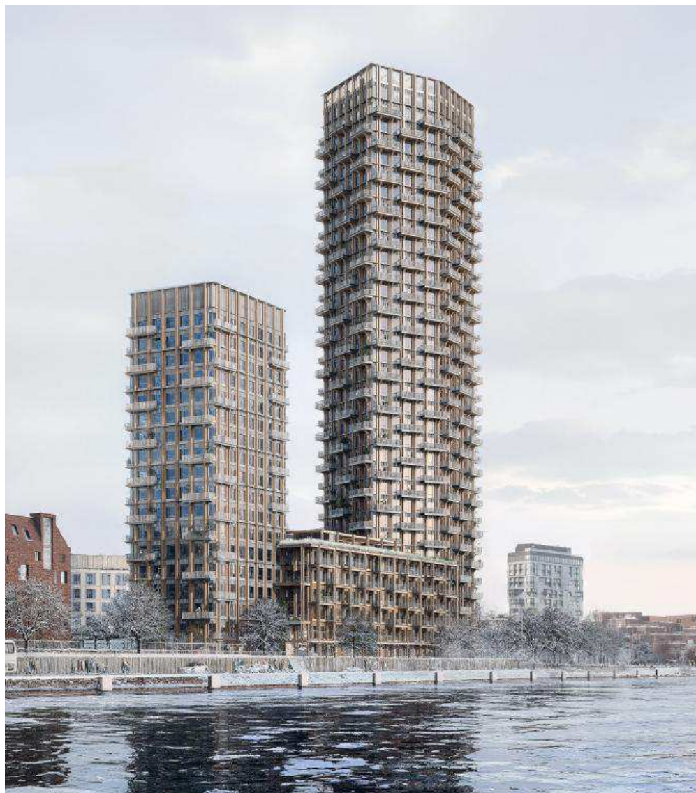
Figur 4-11. Illustration af udnyttelse af lokalplanforslagets byggemuligheder på Langelinie. Lendager, 2026.
