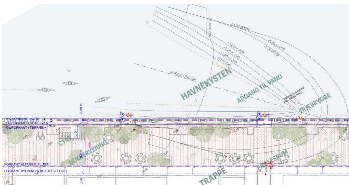
Figur 16-8. Nordic Crown. Påsejling af kaj, Langelinie. Vinkel mellem færge og kaj = 16,2^\circ . Afstand mellem færge og facade er min. 2,10 m.
