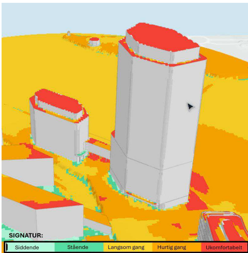
Figur 9-4. Vindkomfortanalyse for området omkring Marmormolen. Set fra vest mod øst. Skalaen viser, hvilken aktivitet, der kan udføres komfortabelt. Rød markering angiver kraftig vind, som er ukomfortabel uanset aktivitetsniveau. Svend Ole Hansen ApS, 2025
