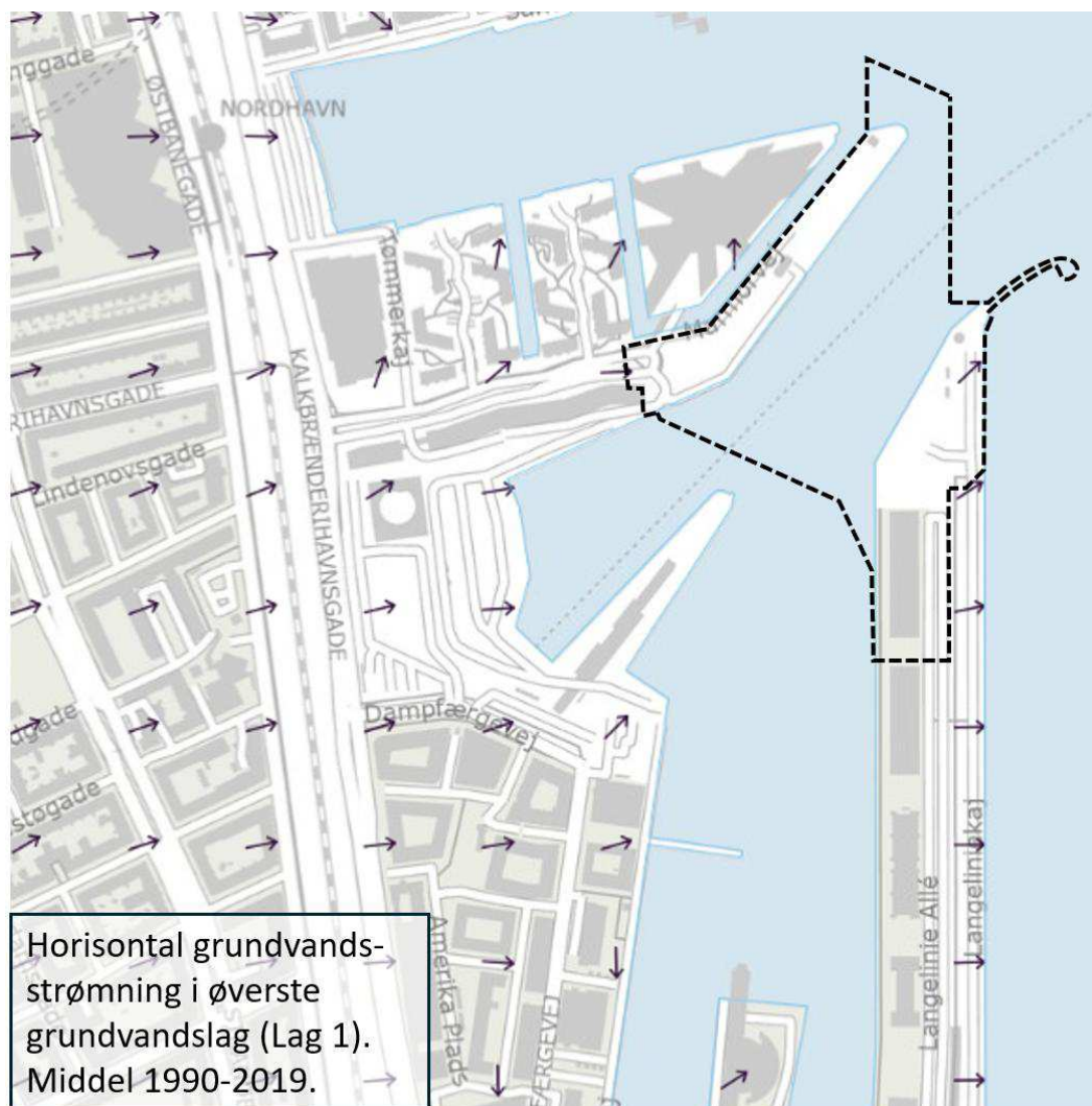
Figur 12-5. Horizontal grundvandsstrømning (middel 1990-2019) i det mest terrænnære lag (Lag 1). Data fra hip.dataforsyningen.dk
