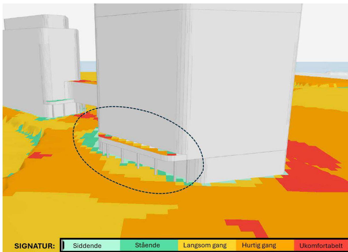
Figur 9-5. Effekten af udhæng over indgangspartiet fra Marmorvej, der beskytter mod downwash. Svend Ole Hansen ApS, 2025
