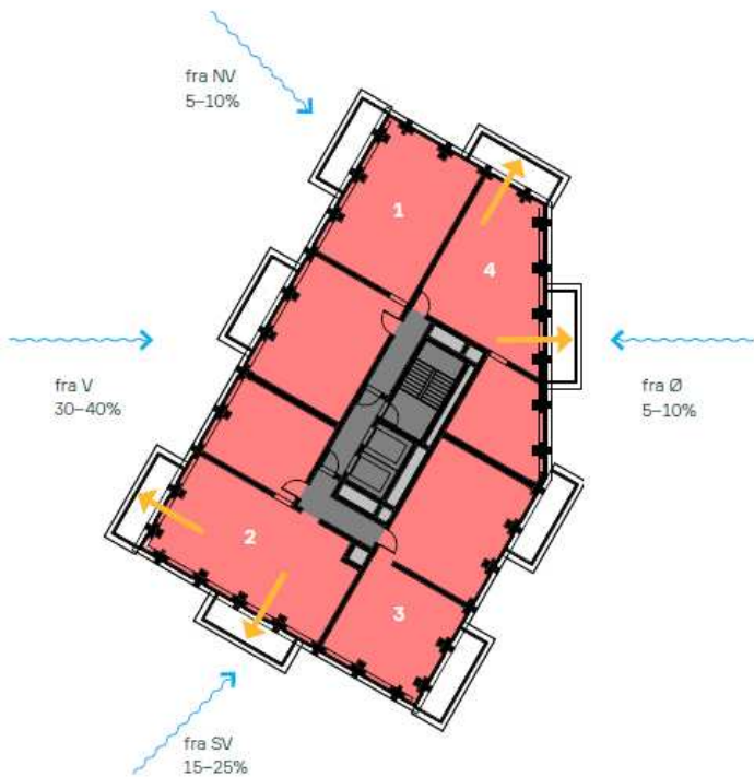
Figur 9-9. Disponering af altaner i to rytmer, der skifter fra etage til etage. Vindretningernes hyppighed angivet med procenttal. Pile inde fra lejligheder angiver mulighed for at tilgå altaner mod to verdenshjørner. Lendager, 2026.
