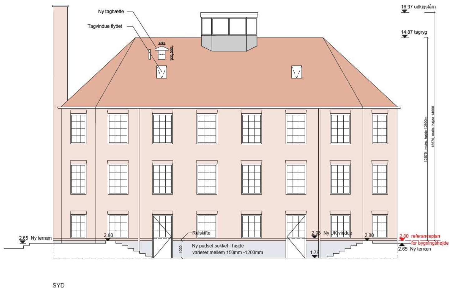
Figur 14-26. Plan over det genopførte Lodseri med angivelse af bygningsmæssige ændringer. Sydfacaden.
