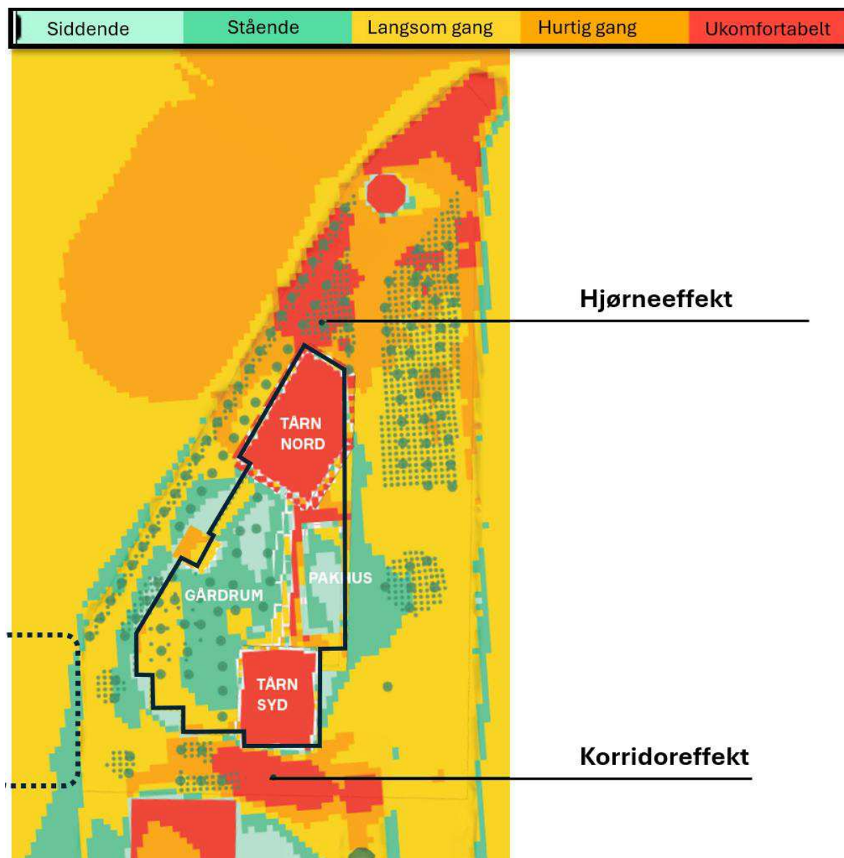
Figur 9-6. Resultat af vindanalyse af byggefelt på Langelinie. Placering af udlæg til mulig mobil badezone markeret med stiplet linje. Lendager, 2026.
