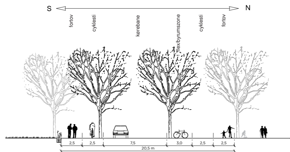
EKSEMPEL PÅ TVÆRSNIT PÅ LILLE TORV
