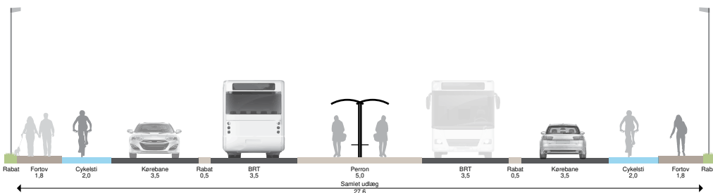
Figur 17 Ø-perron som ved Novembvej. Brugen af Ø-perron reducerer den samlede tværsnit da 2 platforme af 4 m bredde veksles til én central Ø på 5 m. Anvendelse af Ø-perron kræver, at busserne betjener perronen fra venstre kørespor (i kørselsretningen), hvorfor busserne skal krydse fra det ene til det andet spor både før og efter stationen.
