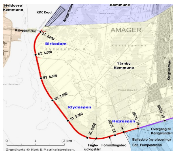
Figur 21: Plantegning af hævning af Vestamager Kystdige, 2012.
