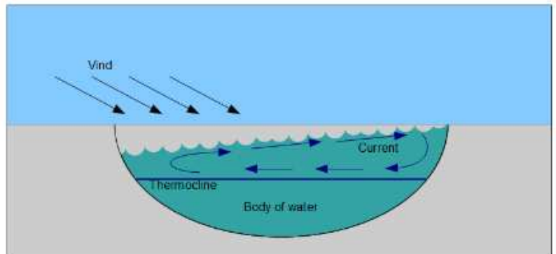
Figur 2: Visualisering af fænomenet seiche (vandstuvning) ved stormflod (Frankemann, 2014)
