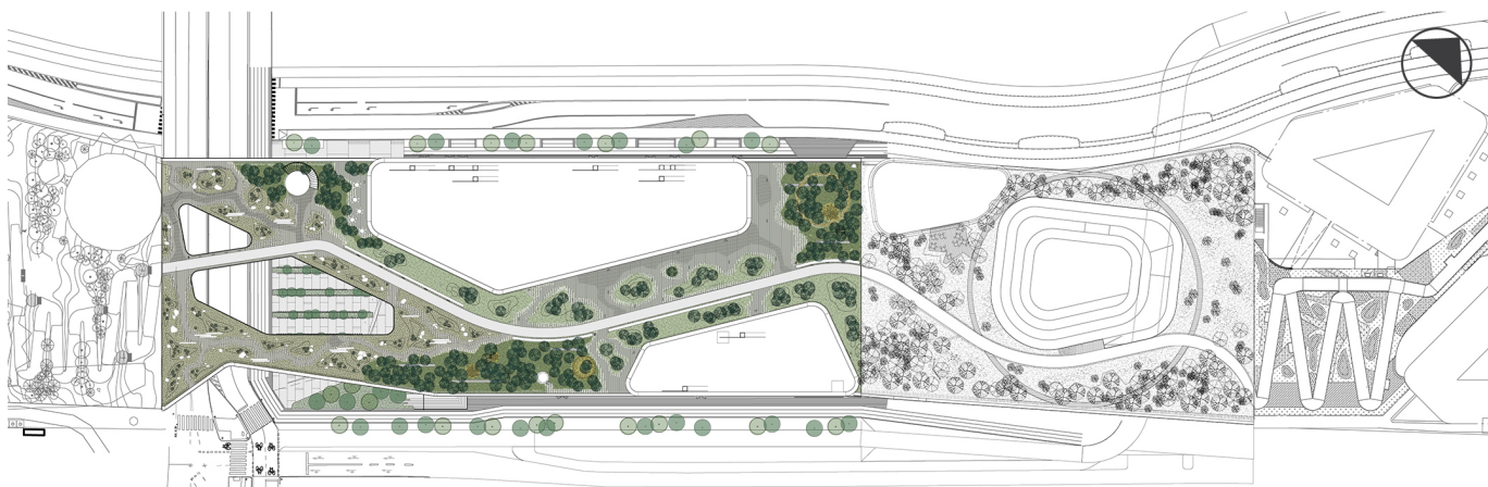
Illustration, der viser taghavens indretning på varehusets tag samt gadetræer langs Carsten Niebuhrs Gade og Kalvebod Brygge. Illustration: 1:1 Landskab.
