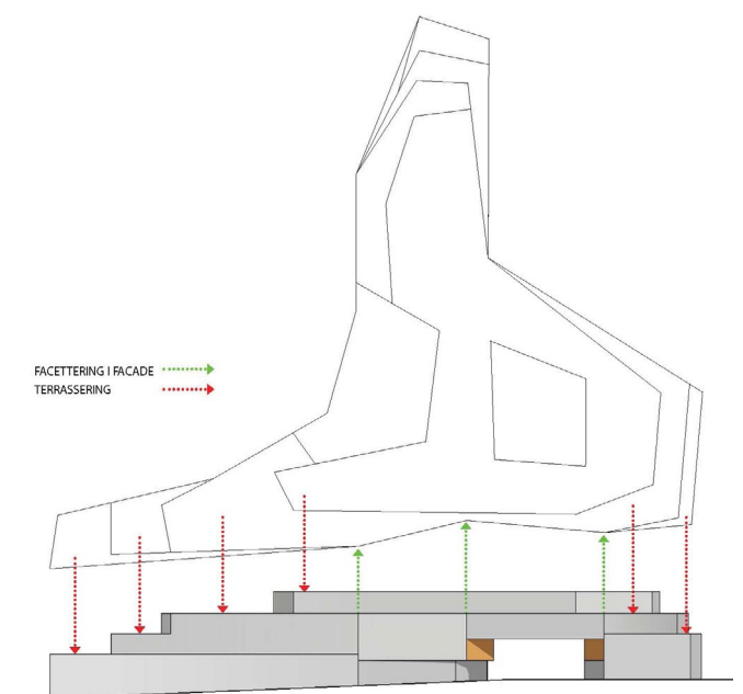
Princip for vinklinger og tilbagetrækninger af facaden som underdeler den lange facade og nedtrapper bygningshøjden mod omgivelserne. Her ses facaden mod Valby Langgade og tagplan. Illustration: C.F. Møller
