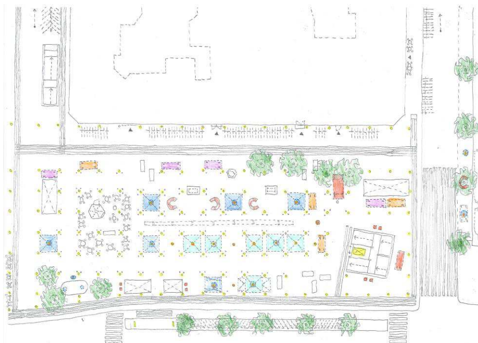
Grundplan af Christianshavns Torv med 18-24 nye stadepladser til fødevarerhandel placeret mellem det lysende gridsystem som definerer hvordan staderne kan opstilles og samtidigt skaber tryghedsskabende lys. Blå stade-enheder er til kød, fisk ost etc. mens grønne stade-enheder er til danske regionale grøntsager, frugter, krydderurter, blomster etc, mens de halve stademoduler typisk er egns-specialiteter, børneboder og gadekøkken. Torvet anbefales desuden funktionelt forlænget ud til Christianshavns Kanal med 2-4 flydende stader via markant bredere fodgængerovergang
