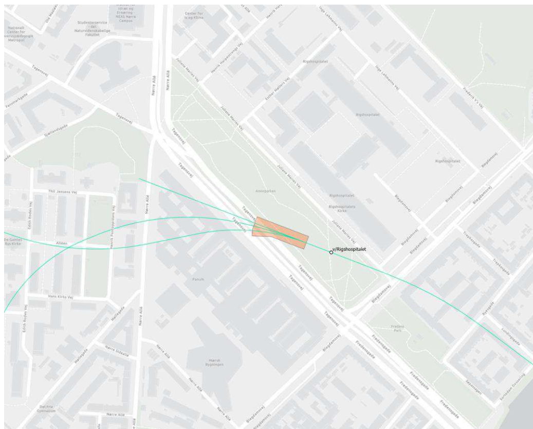
Figur 21: Mulig placering af afgreningsanlæg ved Rigshospitalet.
