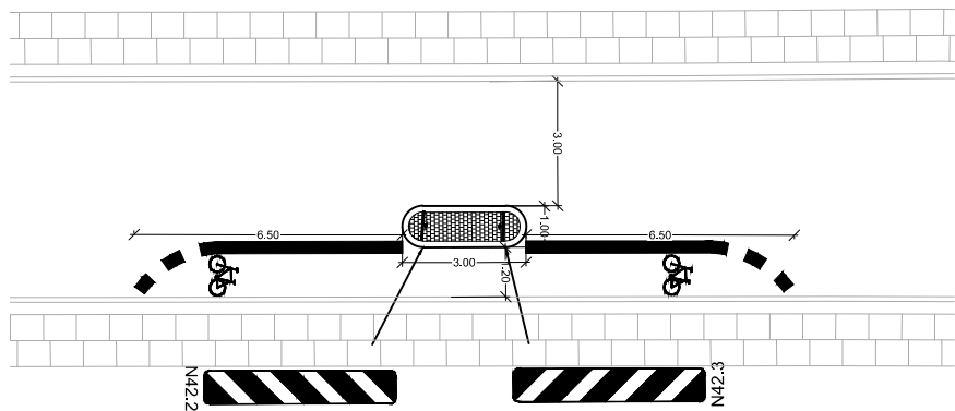
Type 1, Indsnævring til et spor - med cykelsluse
