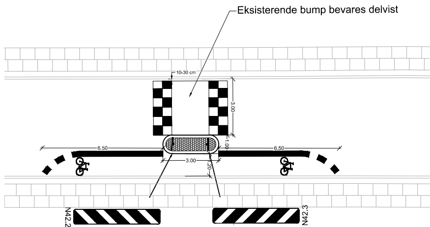
Type 2, Indsnævring til et spor - med cykelsluse og bump
