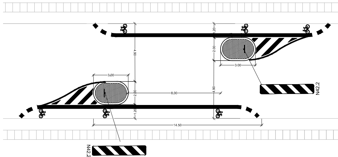
Type 4, Forsætning med indsnævring til et spor - med cykelsluser
