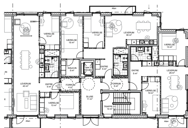
Plantegning 1.-7. sal
