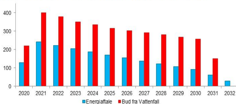
Figur 1. Skønnede årlige PSO-omkostninger til kystnære møller, mio. kr., 2016-priser
