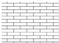
Halvstensforbandt på kant Velegnet til havetegl.
