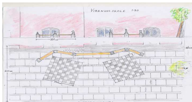
Plan- og opstaltstegning af den samlede installation ved Vibenshus Skoles hovedindgang.
