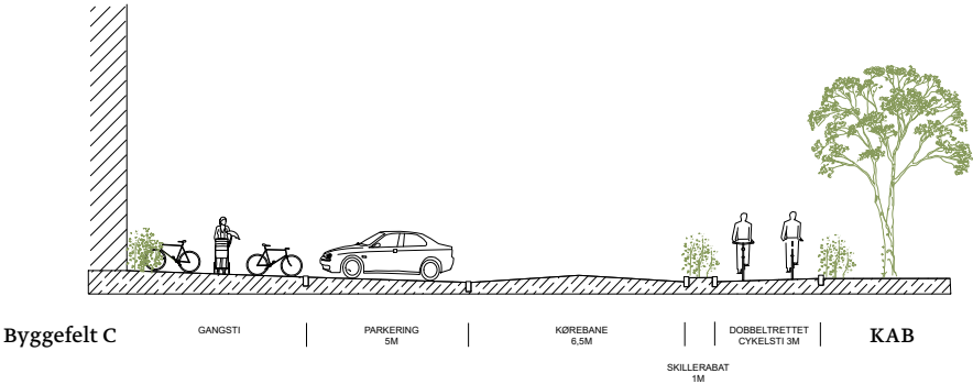
Vejsnit A
