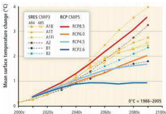
Figur 3: Scenarier for gennemsnitlig temperaturudvikling i forhold til referenceperioden 1986-2005 i RCP-scenarioerne fra IPCC AR5 (2014) og SRES-scenarioerne fra IPCC AR4 (2007) (DMI, 2018)
