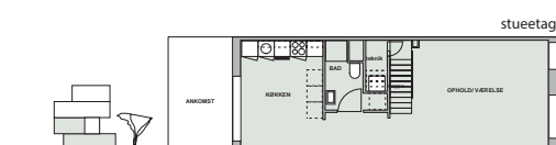
Boligtype 04 - 82m 2 - adgang fra stueetage
