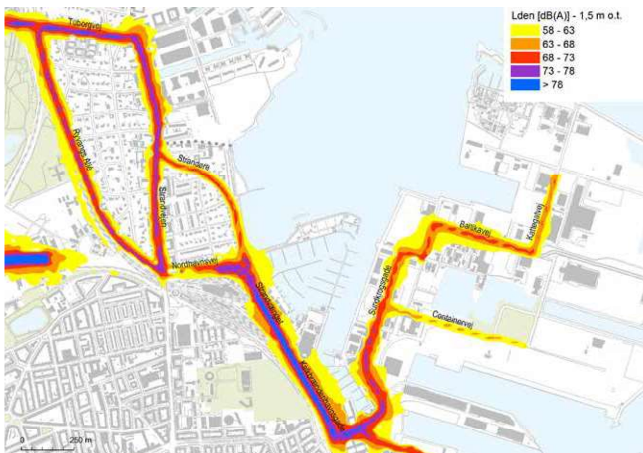
Figur 9.17 Støjniveaukonturer, 0-alternativ.
