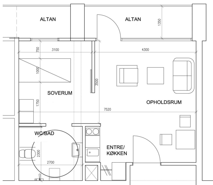
Bygning 3 møbleringsplan boligtype 3-01 1:100
