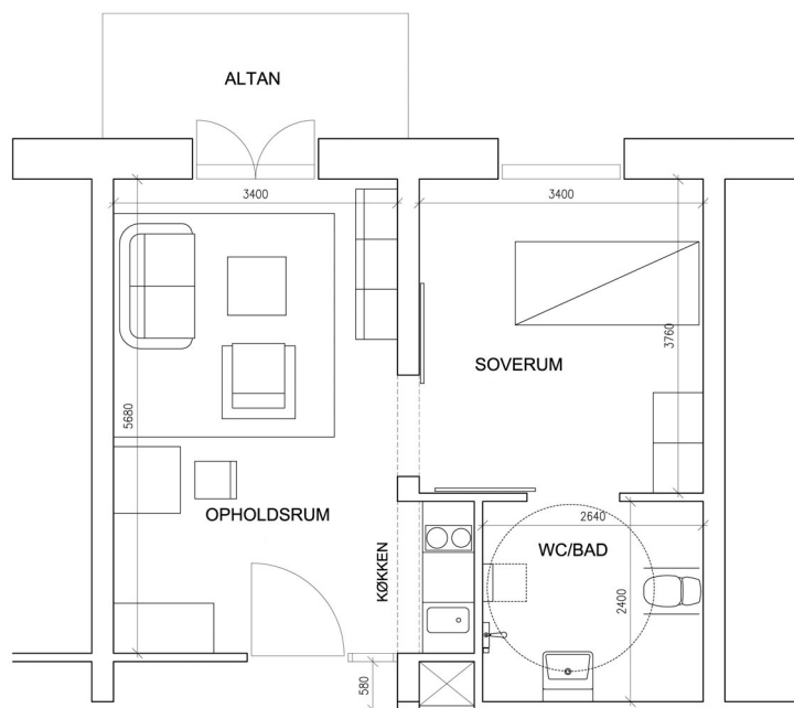
Bygning 1 møbleringsplan boligtype 1-01 1:100
