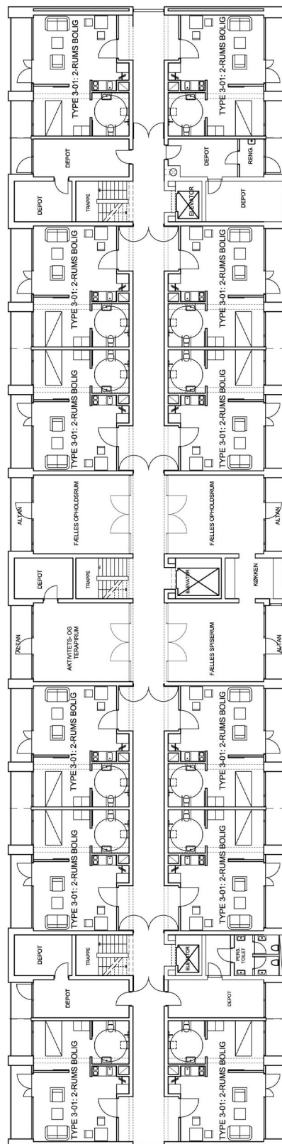
Bygning 3 plan 1.-3. Sal
