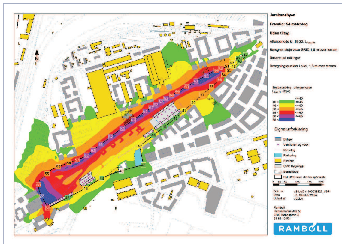
Figur 19-3. Scenario: Uden støjdæmpende tiltag. Beregnet støjniveau i skel og støjkontour 1,5 meter over terræn i aftenperioden.
