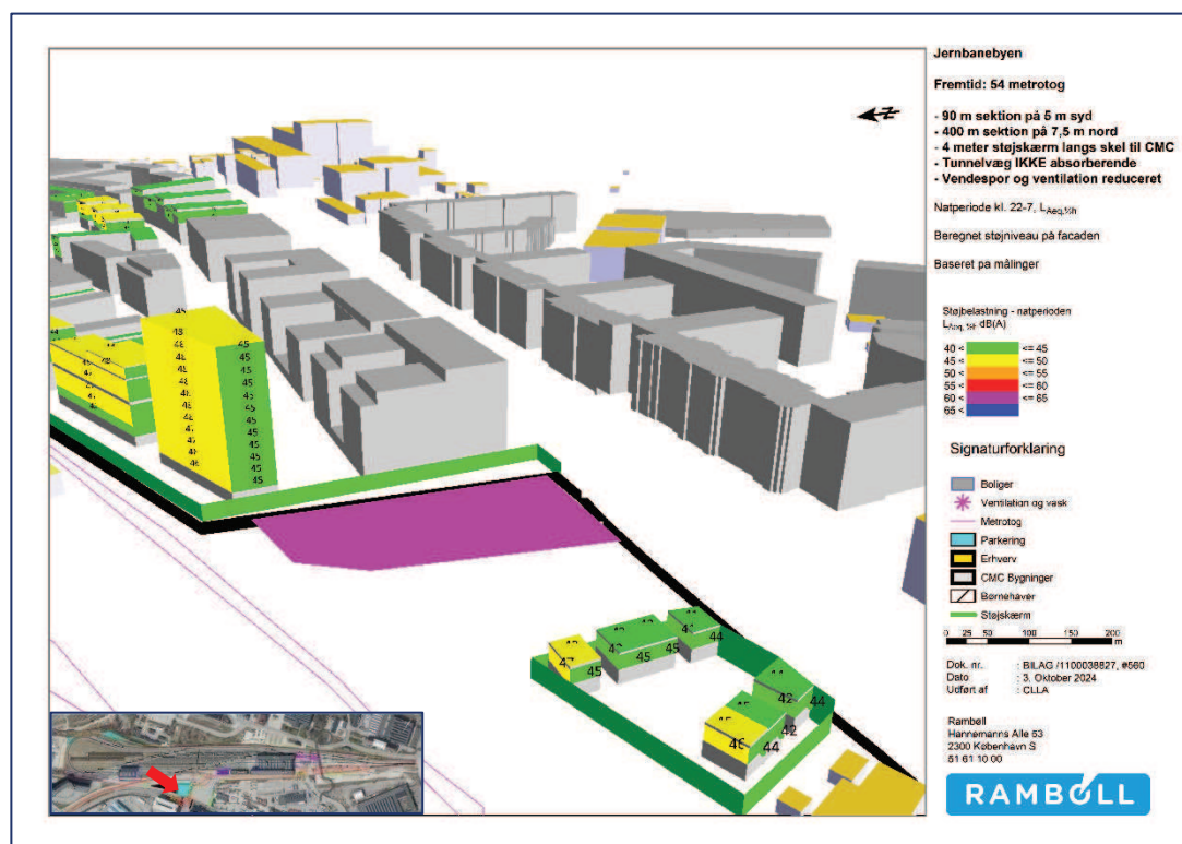
Figur 19-27. Scenarie: Reduceret støj uden overdækning. 3D opstalt af beregnet støjniveau på facaden i natperioden. Grå facader er udsat for støj med niveauer under 40 dB. Bygninger på sydøst side midt for CMC.
