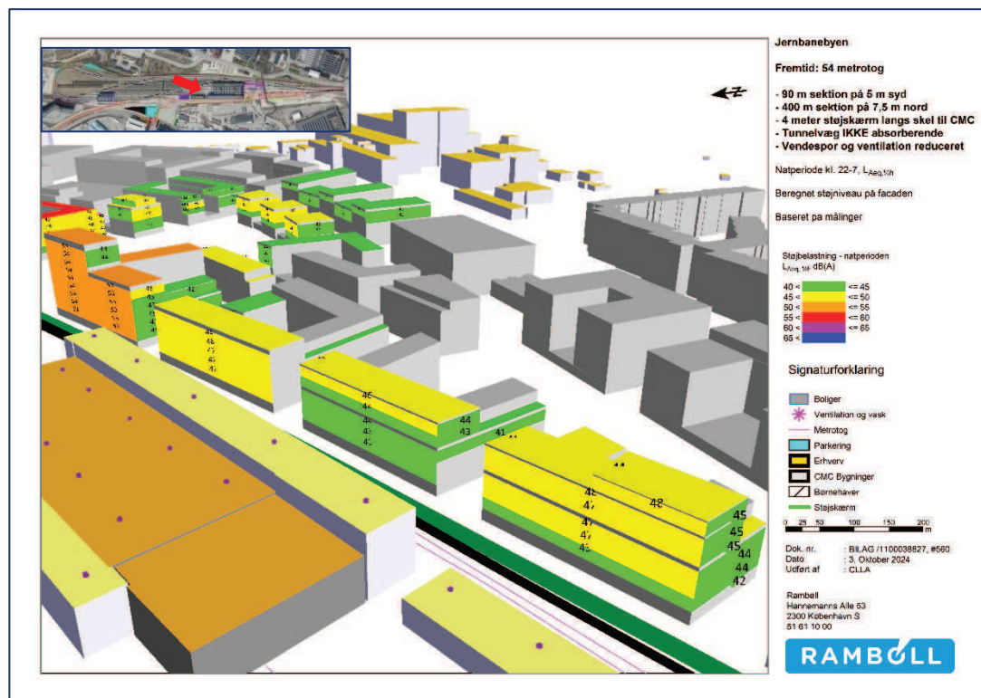
Figur 19-28. Scenarie: Reduceret støj uden overdækning. 3D opstalt af beregnet støjniveau på facaden i natperioden. Bygninger på sydøst siden ud for CMC værkstedsbygning.
