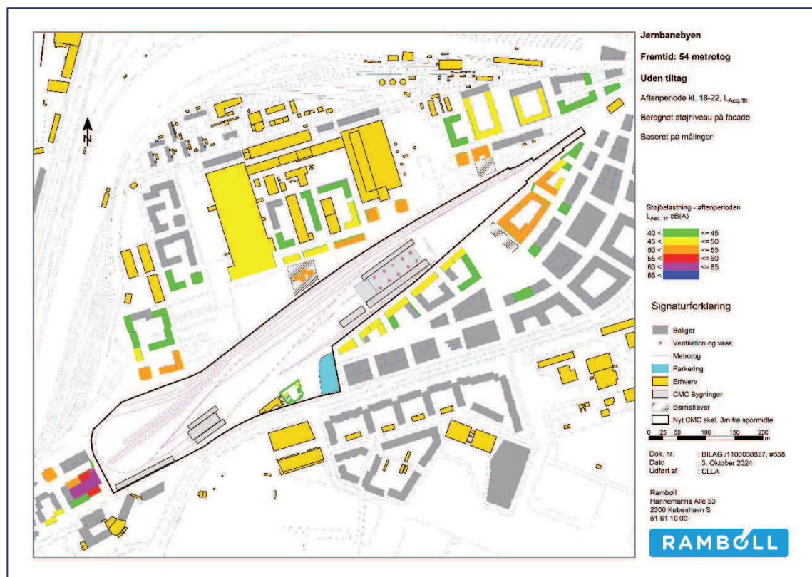
Figur 19-4. Scenario: Uden støjdæmpende tiltag. Beregnet støjniveau på facaden i aftenperioden. Grå bygninger er udsat for støj med niveauer under 40 dB.
