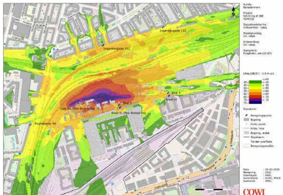
Figur 3 Støjdbredelseskort for Kulgården - nuværende forhold.
