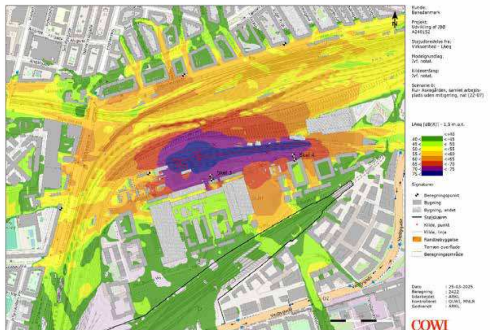
Figur 5 Støjbreddes kort for fremtidig samlet arbejdsbase i Askegården, uden støjmitigerende tiltag.
