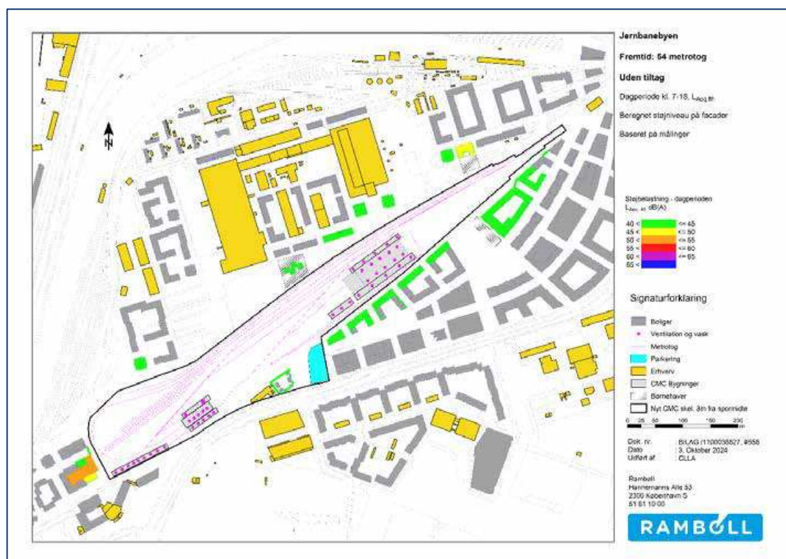
Figur 20-2. Scenarie: Uden støjdæmpende tiltag. Beregnet støjniveau på facaden i dagperioden. Grå bygninger er udsat for støj med niveauer under 40 dB.
