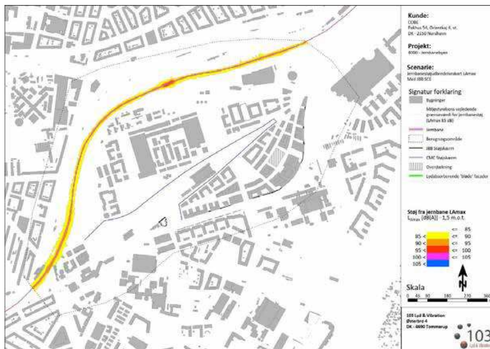
Figur 10-18 Støjdbredelseskort støj L_{max} fra jernbane 1,5 meter over terræn for fremkrevet scenario år 2032 (103).
