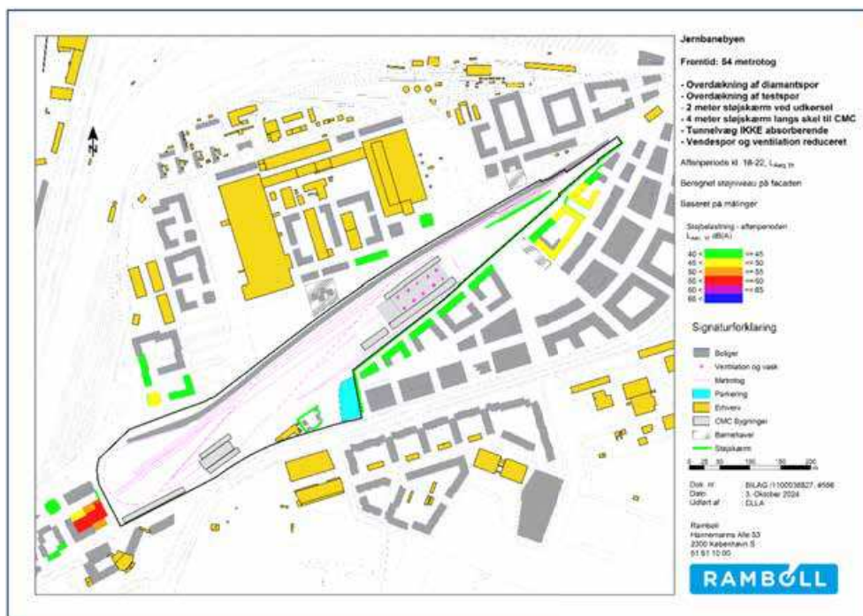
Figur 6-12 CMC. Støjdæmpende tiltag i form af overdækning når planlovens § 15, stk. 2, nr. 29, jf. § 15a, stk. 1 finder anvendelse. Facadestøjskorte aftensperioden (Rambøll).
