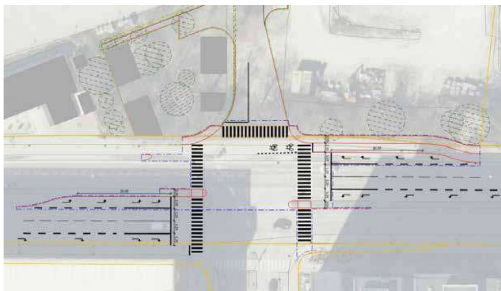
Figur 3-6 Foreslået krydsudformning for det signalregulerede kryds ved Vestre Teglgade/Vasbygade. Det sidste tilføjede ben mod nord vil kun håndtere trafik til/fra CMC. Krydsudformningen anvendes i Scenario 2035.
