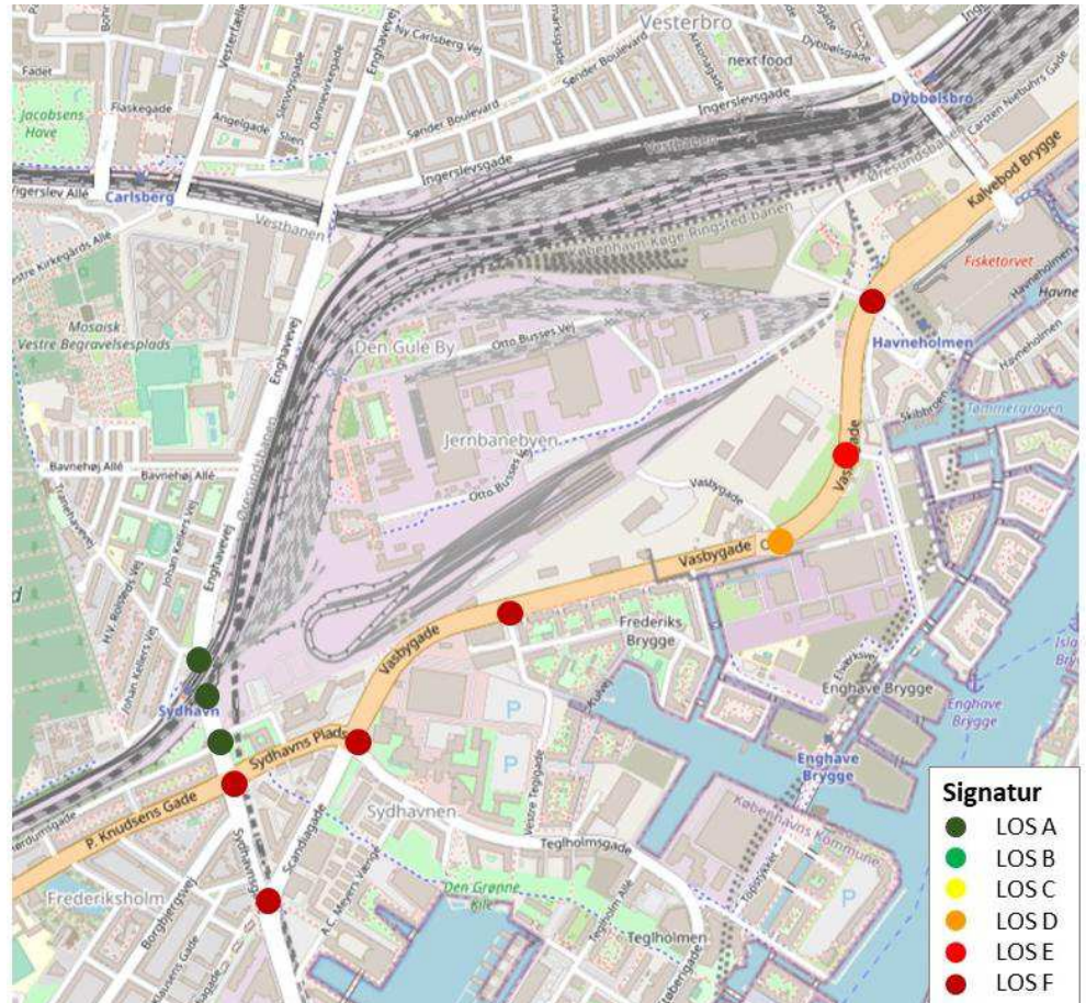
Figur 5-7 Beregnet serviceniveau (LOS) af de undersøgte kryds i Basis 2035 i eftermiddagsmyldretiden (kl. 15-17). Definitionen af serviceniveauer er angivet i tabel 5-1.
