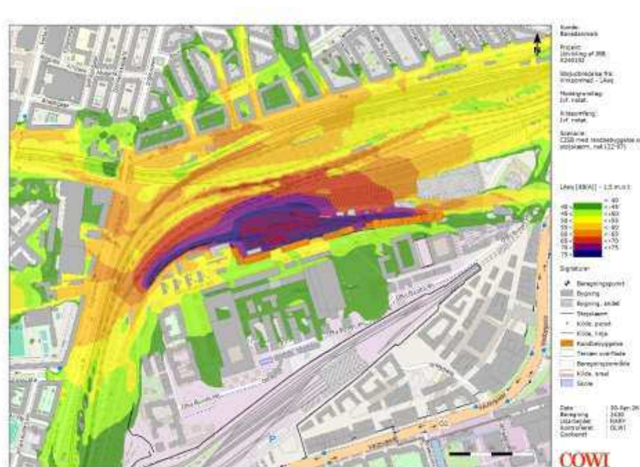
Figur 5 Støjudbredelseskort for CISB fremtidige forhold – natperioden.
