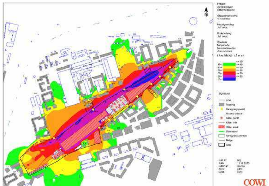
Figur 5-9 CMC. Støjuddbredelseskort uden støjdæmpende foranstaltninger ved fuld udnyttelse af støjvilkår (COWI). (Beregningerne er ikke foretaget på det mest opdaterede bygningslayout).
