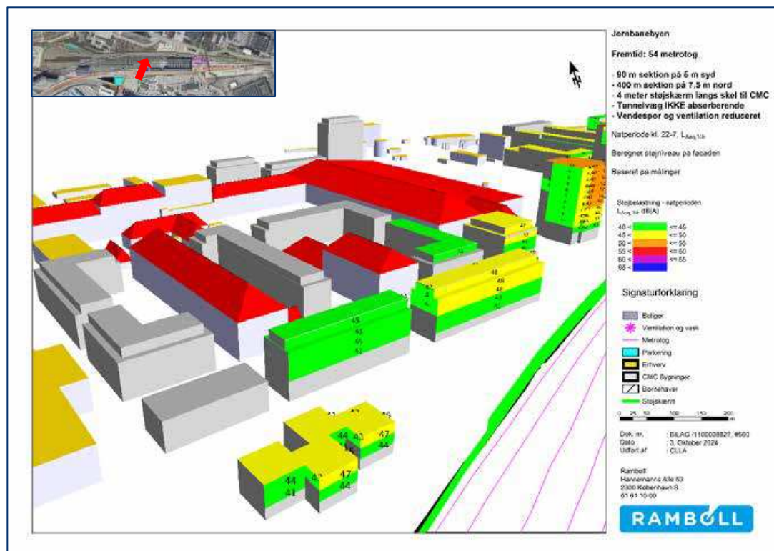
Figur 20-24. Scenarie: Reduceret støj uden overdækning. 3D opstalt af beregnet støjniveau på facaden i natperioden. Grå facader er udsat for støj med niveauer under 40 dB. Bygninger ved Lokomotivværkstedet nordøst for CMC.
