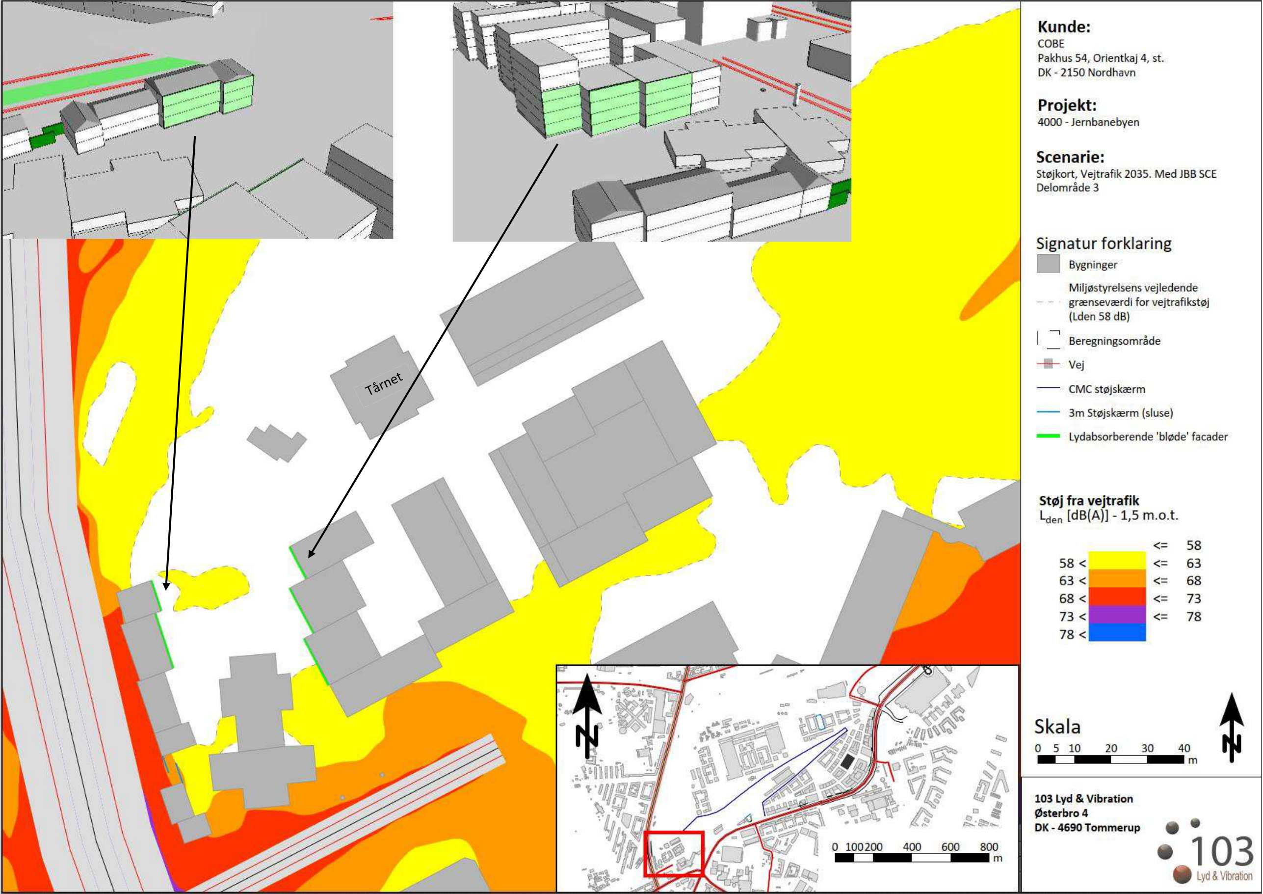
Beregningsresultater i Delområde 3 – Vejtrafik-støjudbredelseskort i 1,5 m over terræn
