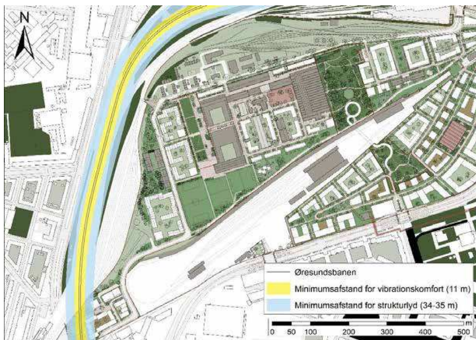
Figur 6 Minimumsafstand for at acceptabelt niveau for vibrationskomfort og strukturlyd for bolig- og erhvervsbyggeri tæt på Øresundsbane for hastigheden på strækningen 120 km/t (fjernest Københavns Hovedbanegård) og 70 km/t (nærmest Københavns Hovedbanegård).
