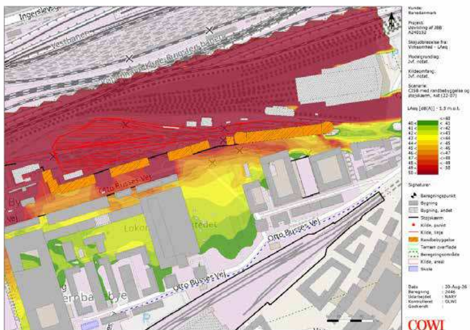
Figur 1. Delområde 5 og 6. Byggnadsfacader, for hvilke akustisk absorption beregningsmæssigt er etableret, er markeret med rød stiplede linje.
