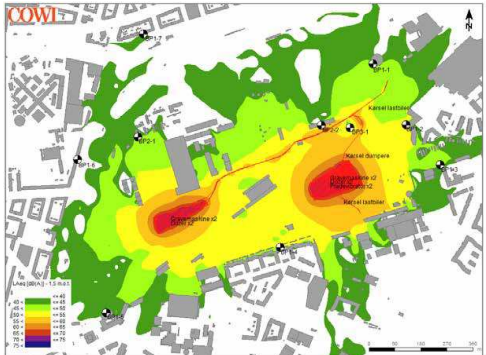
Figur 10-8 Støjudbredelseskort, Scenarie 2 – Terrænregulering. (Kort: COWI).
