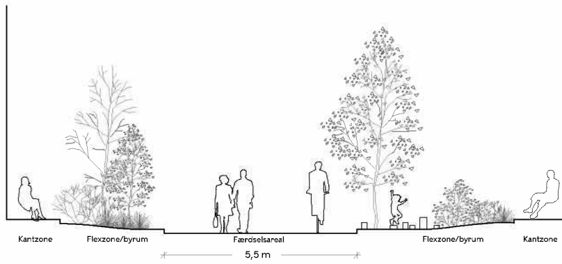
Snit C1
