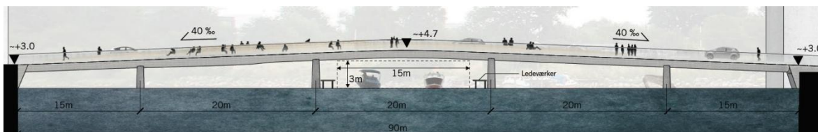
Figur 8: Opstalt af broen (Udsnit fra tegning VB440-1-01-04)
