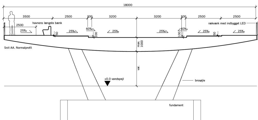
Figur 9: Normaltværsnit af broen (Udsnit fra tegning VB440-3-01-07)
