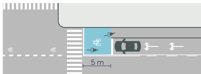
Figur 25: Cykelboks i T-kryds
