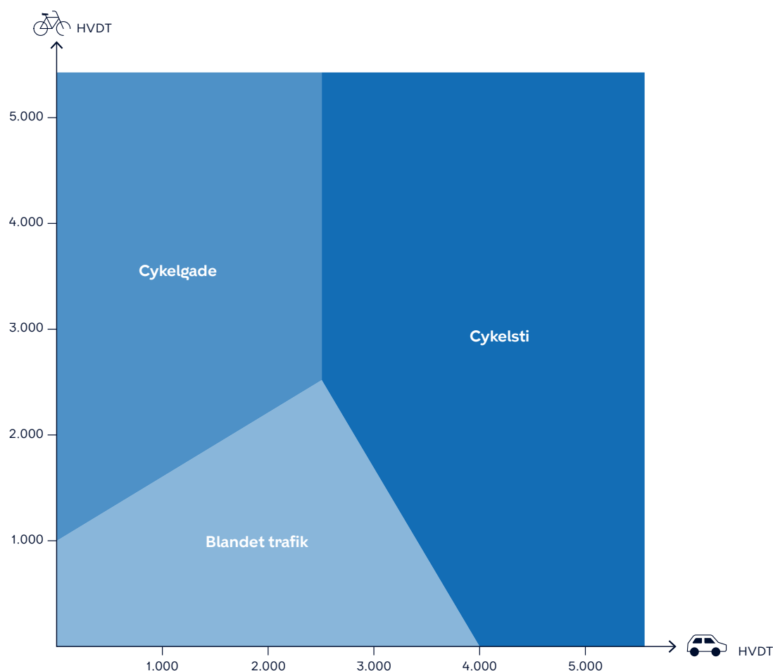
Figur 1 Vejledning til cykelinfrastruktur i sammenhæng med trafikmængder
