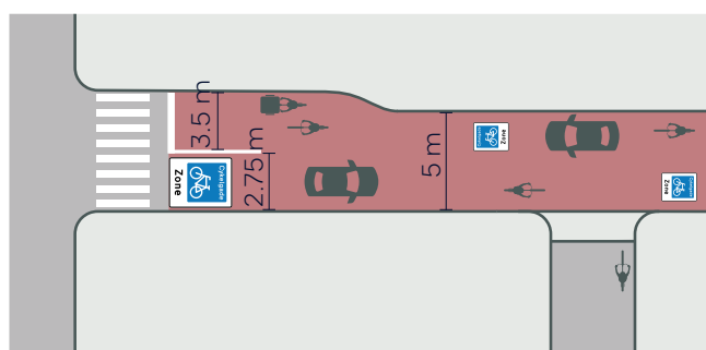
Figur 6: Smal cykelgade uden midterlinje
