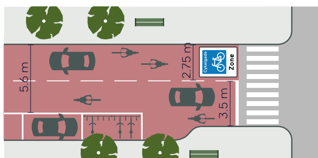
Figur 7: Cykelgade med fortovsudvidelse, cykel- og bilparkering
