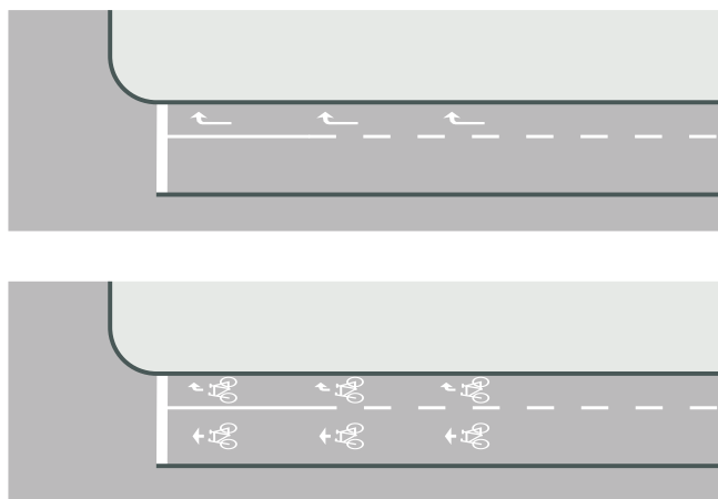
Figur 10: To måder at afmærke kanalisering på cykelstien
