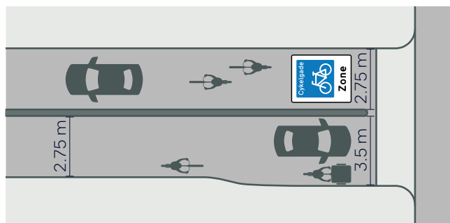
Figur 5: Cykelgade med overkørbart brostensbånd
