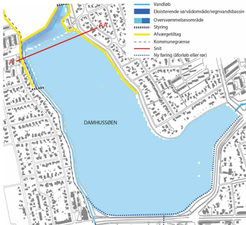
Figur 33 Principplan oversvømmelsesareal delprojekt ID 1.12.2
