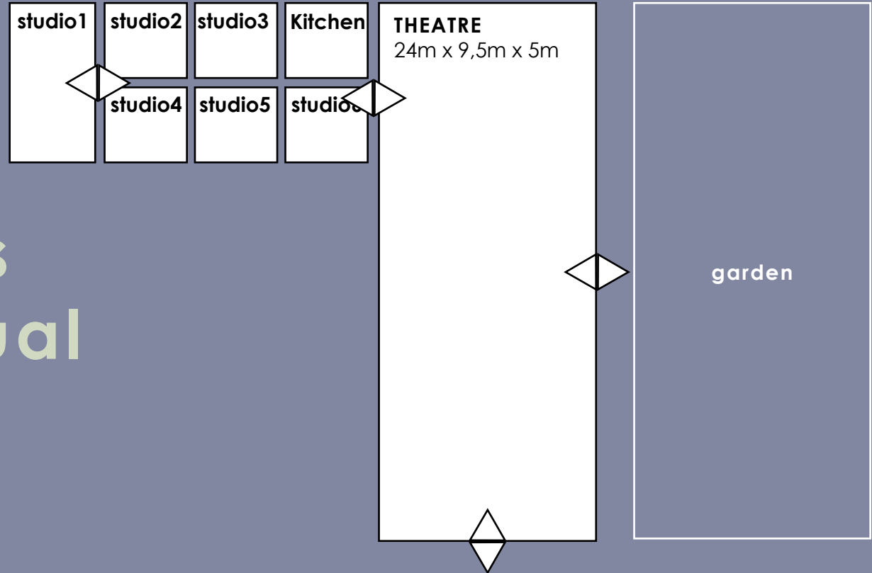
kasernen / groundfloor
