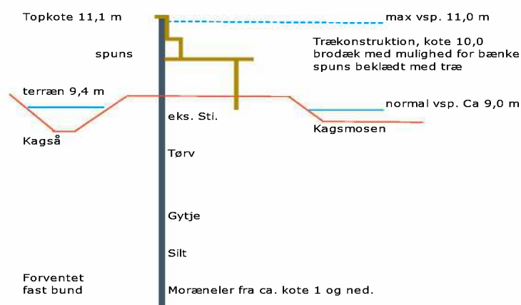
Figur 3-22 Principskitse af mulig konstruktion, baseret på spuns og trækonstruktion, med delvis hævet løsning.
