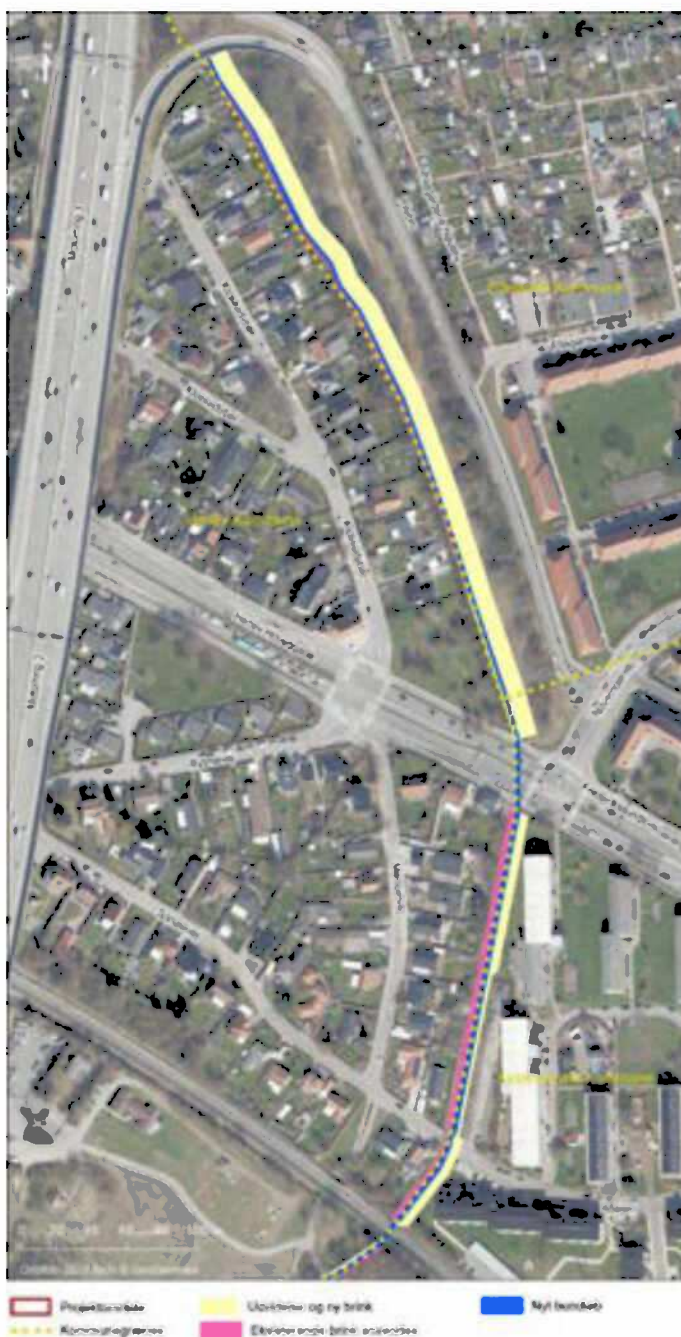
Figur 3-4 Udvidelse af Kagsåen fra Motorring 3 til Herlev Hovedgade og fra Herlev Hovedgade til jernbanen.
