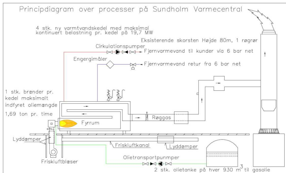
Figur 4 Principdiagram over produktionsprocessen ved oliefyring.
