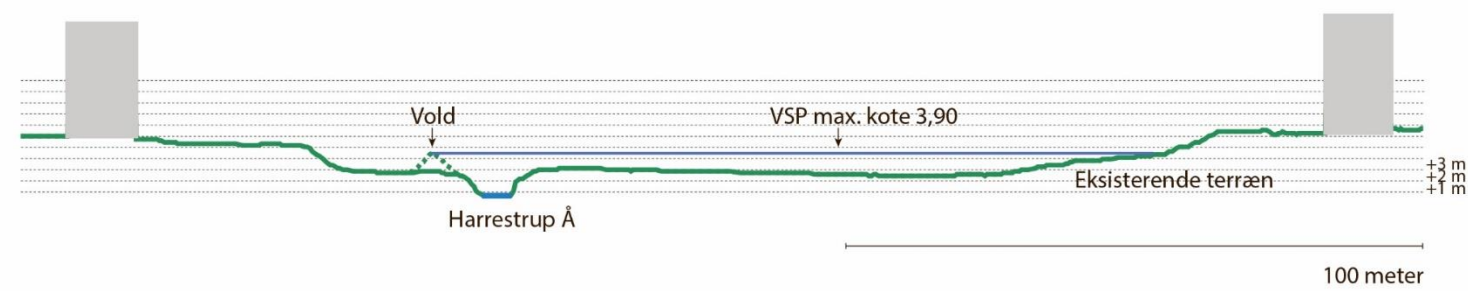
Tværsnit af oversvømmelsesareal ved Vigerslevparken 2 (højde er overdrevet)
