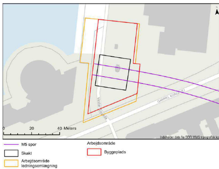
Figur 4.75 Arbejdsområde for ledningsmægninger ved Vester Søgade.
