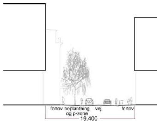
Snit B-B
