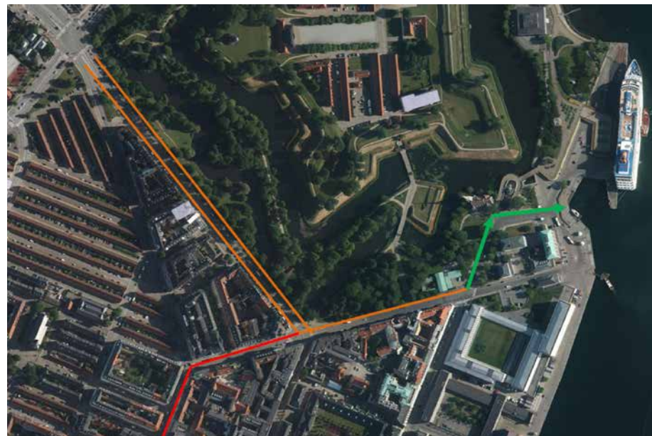
Fig. 3 Forslag til nedgravet og lukket kanal under cykelsti i Grønningen og Esplanaden
