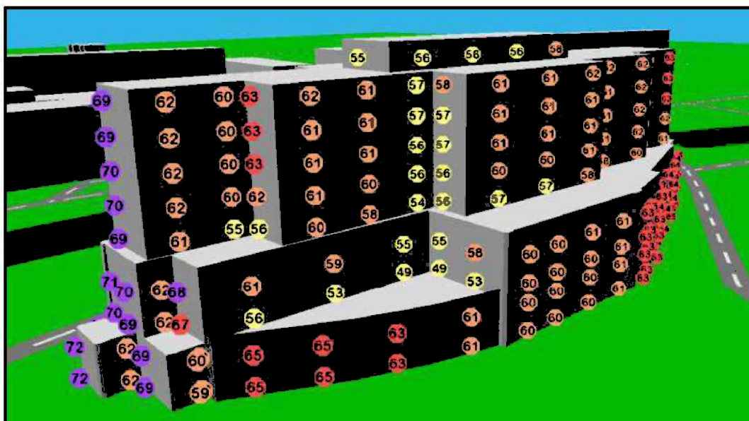
Figur 12.5: Støjniveauer for vejstøj ( L_{den} ) på syd- og østvendte facer mod Axeltorv. ©Buro Happold
