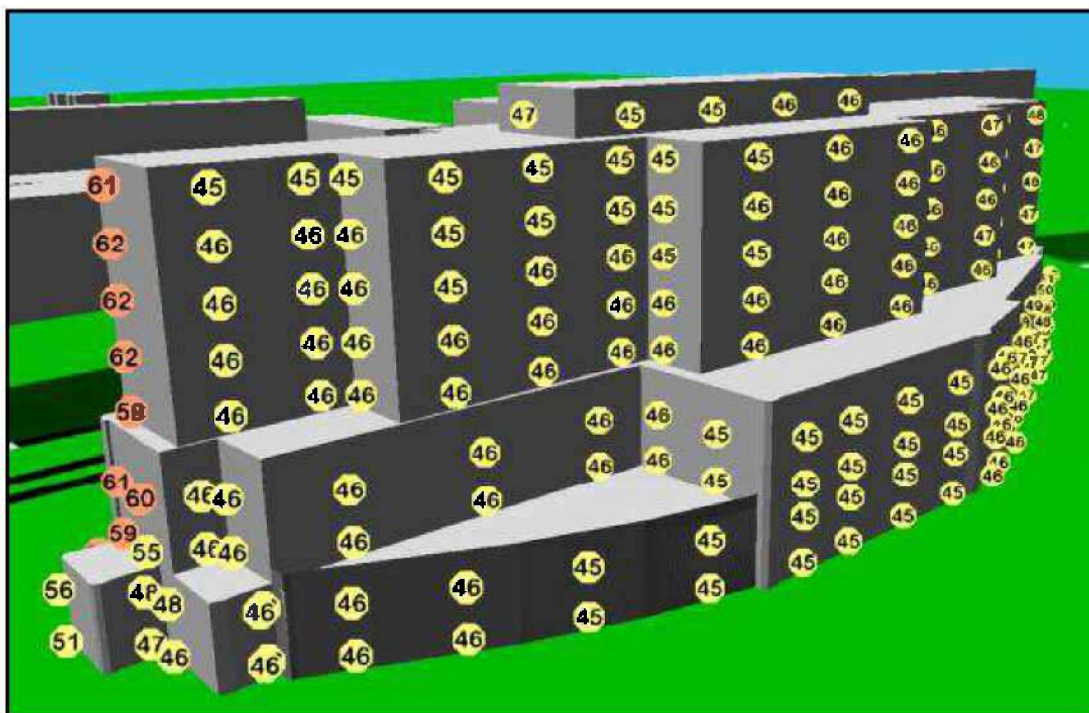
Figur 12.8: Støjniveauer for jernbanestøj ( L_{den} ) på syd- og østvendte facer mod Axelstorv. ©Buro Happold
