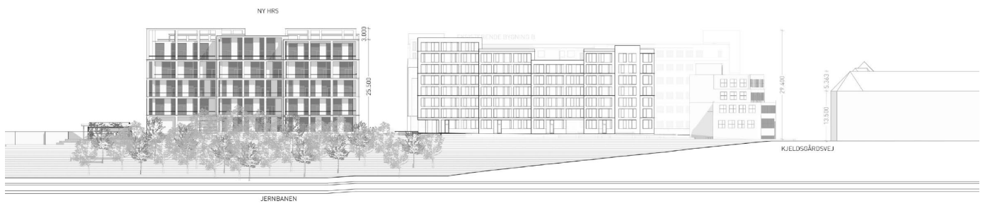
Opstalt set fra nord (jernbanen), der viser et eksempel på et nybyggeri i overensstemmelse med lokalplanen. Illustration: Juul Frost Arkitekter.
