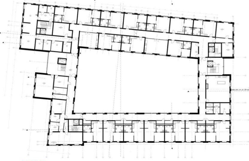
STUEPLAN (og 1.)
