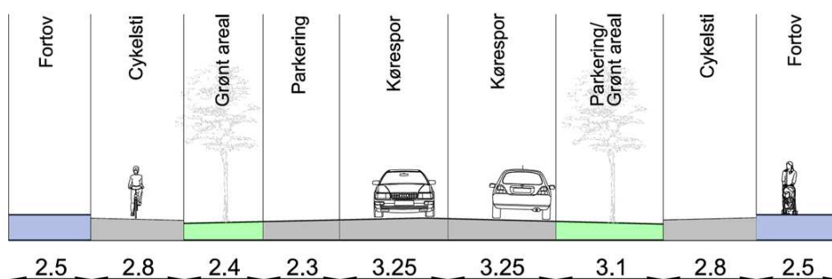
Figur 4: Tværprofil forslag 1
