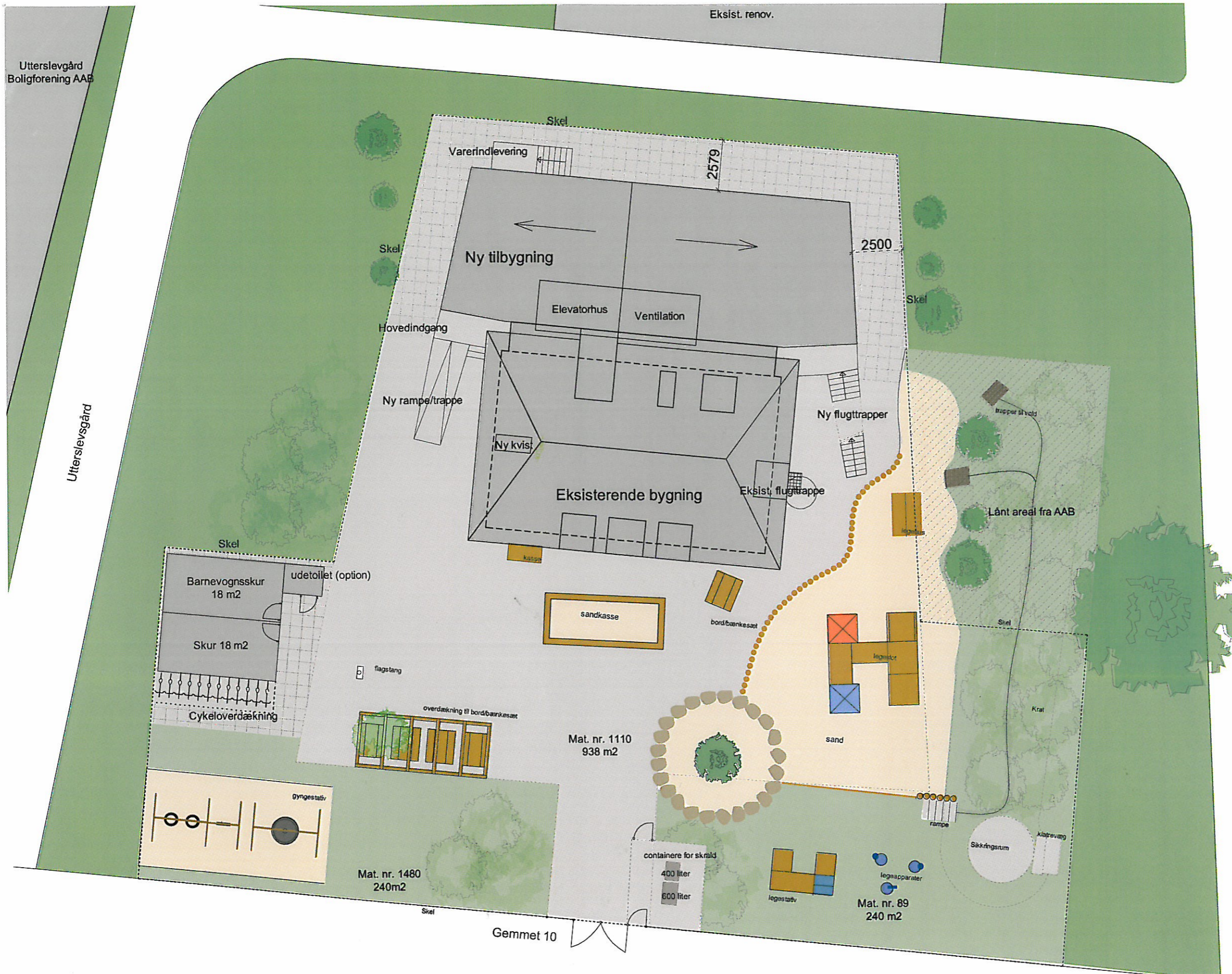
Situationsplan 1 : 200
