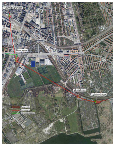
Figur 1. Valby Skybrudstunnel – tunneltracé og skaktplaceringer.
