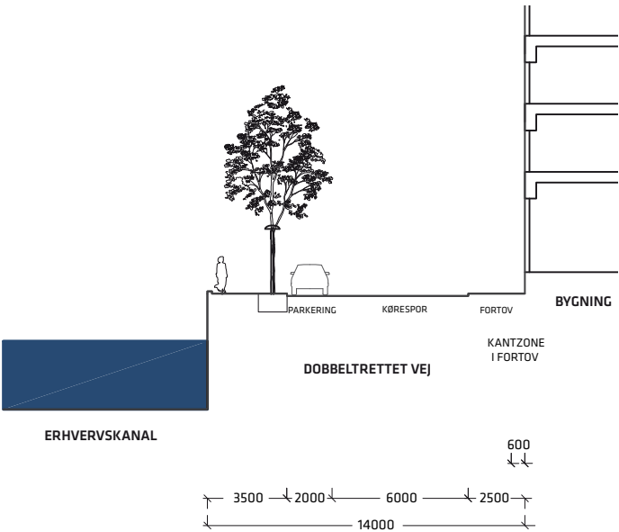
Snit A-A
