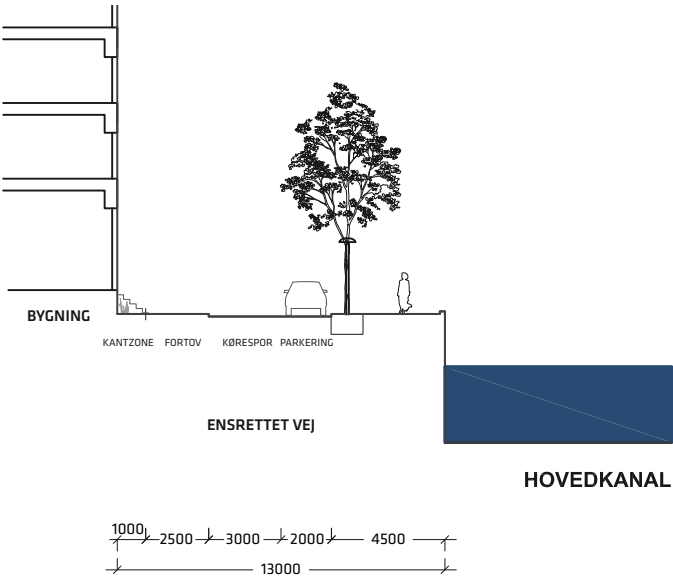
Snit B-B
