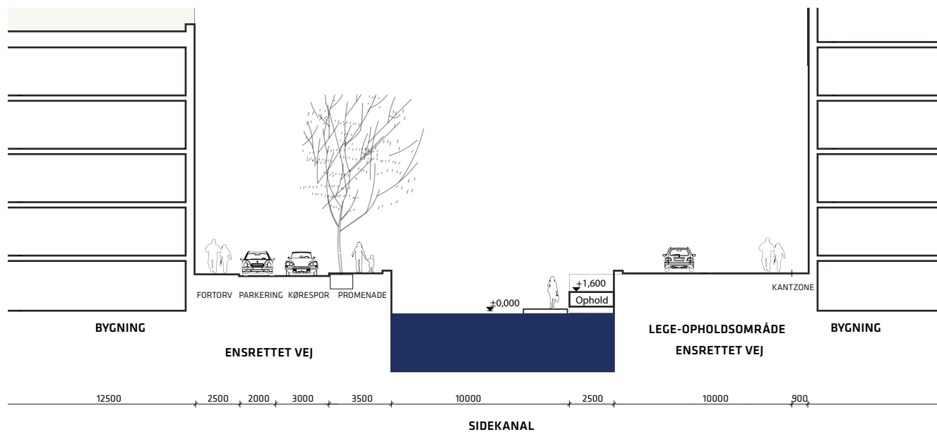
Snit M-M
