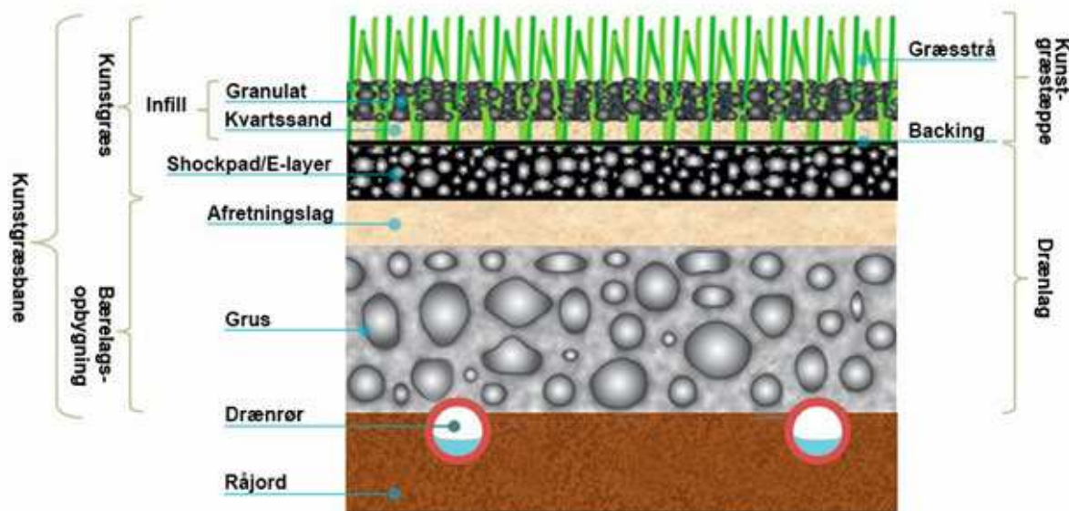
Figur 11-1 Principsskitse for opbygning af en 3. generations kunstgræsbane. Kilde: Vejledning om kunstgræsbaner (Miljøstyrelsen 2018)
