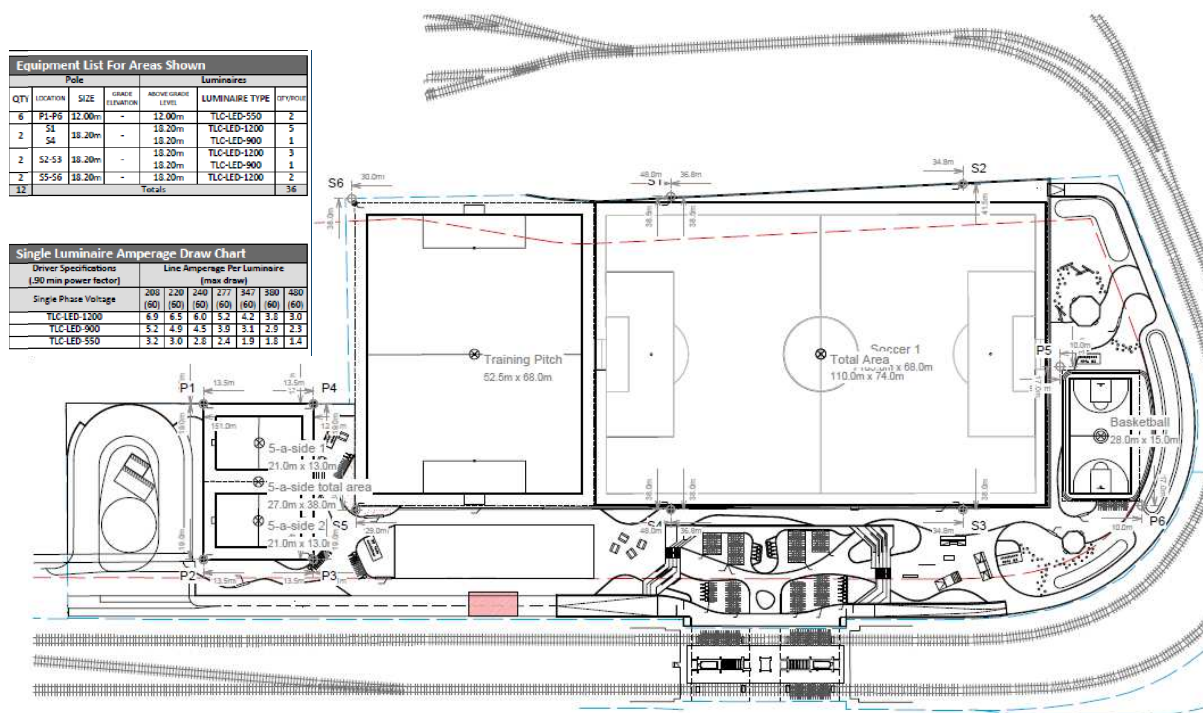
Figur 7-1 Placering af master, højder og udstyr. Kilde: Luma Lysteknik/Musco, se også Bilag 2.
