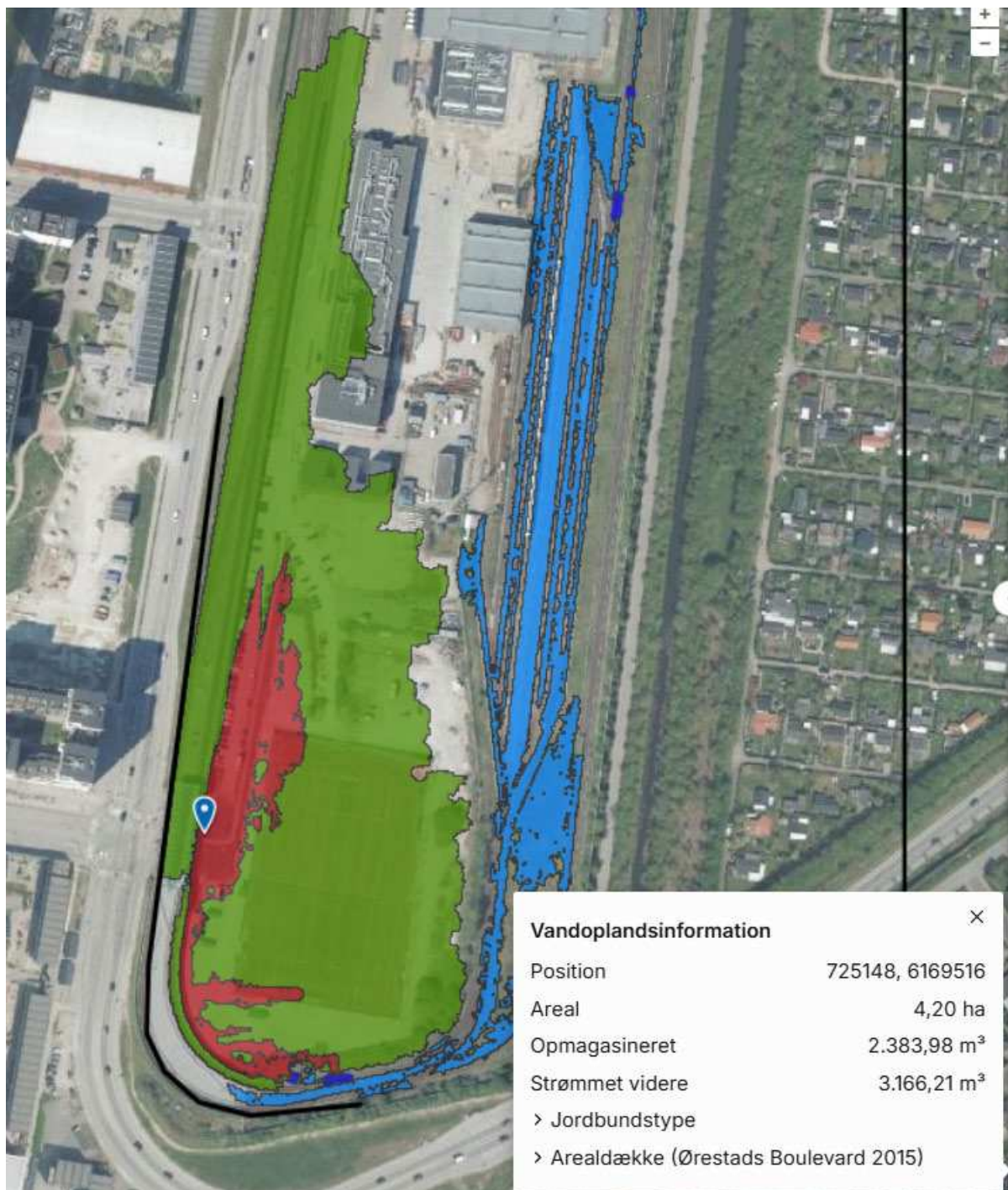
Figur 10-3 Skybrudsopland isoleret til den østlige side af metropassagen i Scalo. Dybdepunkt er vist med rød. Opland er vist med grøn. Kilde: Scalgo/Artelia.
