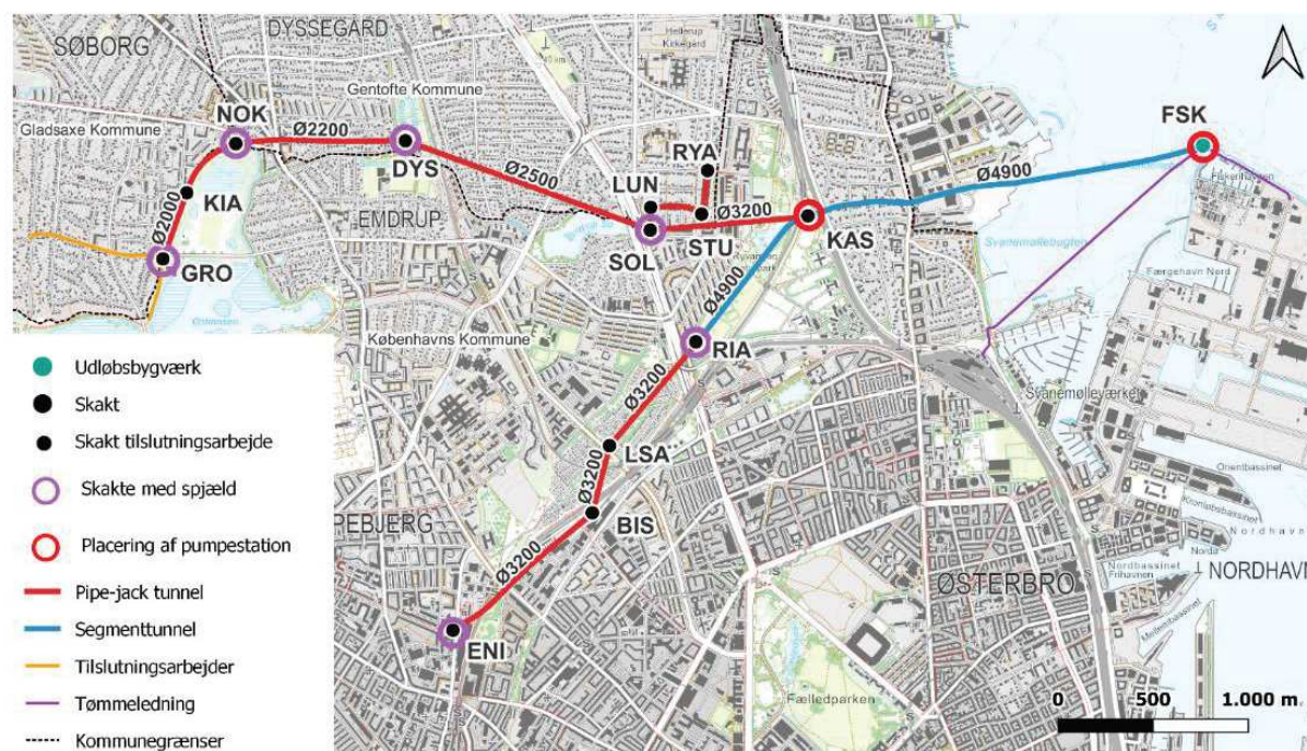
Figur 1: Tracé for Svanemøllen Skybrudstunnel
