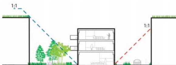
Fig. 5.1 jf. stk. 3. Illustrationen viser at højdegrænsplanen på 1:1 overholdes mod en side i forhold til bygningen i midten
